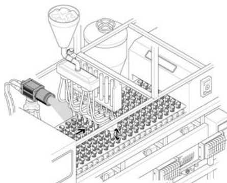
Przykład zastosowania SBOx-Q – proces napełniania.
