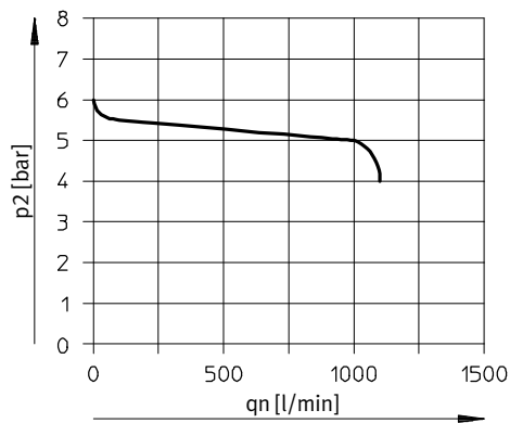
Filterfeinheit 5 µm
