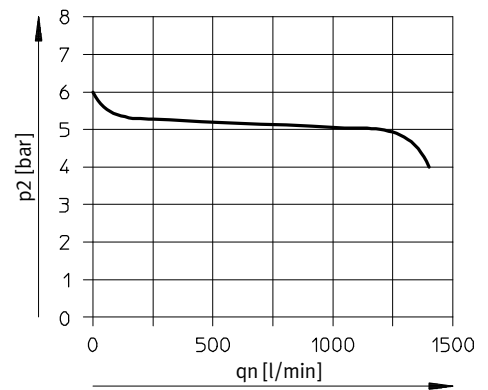
Filterfeinheit 40 µm
