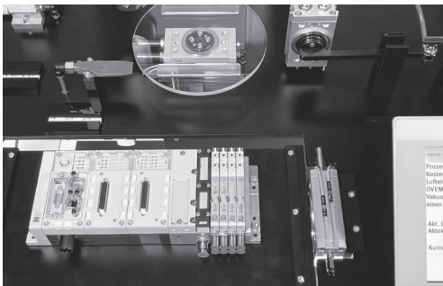
Standardlösung mit Ventilinsel MPA und Kraftregelung über Achscontroller CPX-CMAX.
