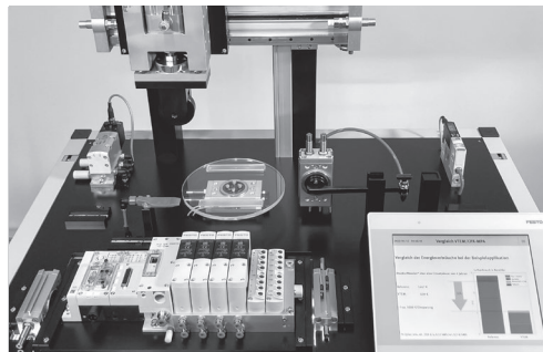
Energieoptimierte Lösung mit Motion Terminal VTEM und den Motion Apps: „Wählbares Druckniveau“, „Zu- und Abluftdrosselung“, „Positionieren“, „Proportional-Druckregelung“.
