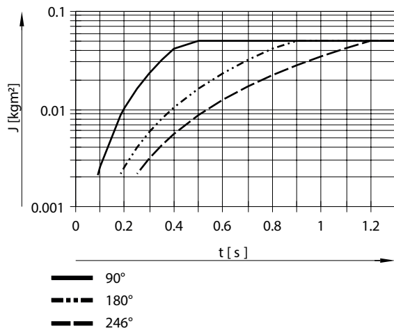
Massenträgheitsmoment J in Abhängigkeit von Schwenkzeit t mit Dämpfung CC für DSM-32
