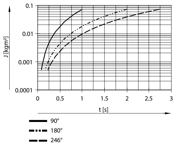
Massenträgheitsmoment J in Abhängigkeit von Schwenkzeit t mit Dämpfung P1 für DSM-32
