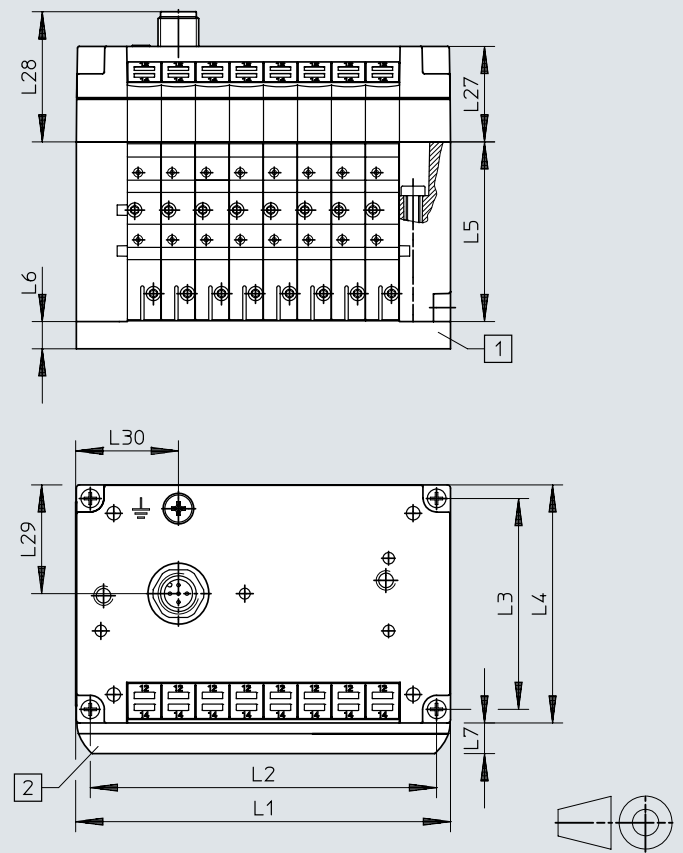
Ventilinsel mit I-Port Schnittstelle/IO-Link – CPV10/14
