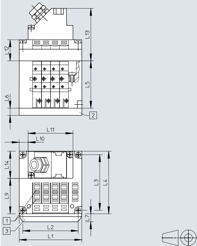
Ventilinsel mit Multipolanschluss – CPV10/14/18
