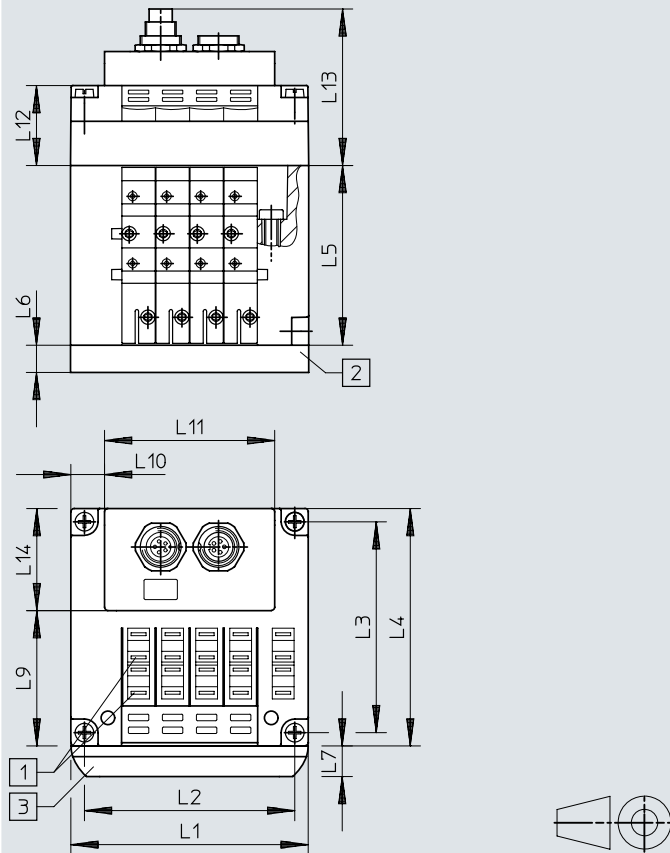
Ventilinsel mit Installationssystem CPI – CPV10/14
