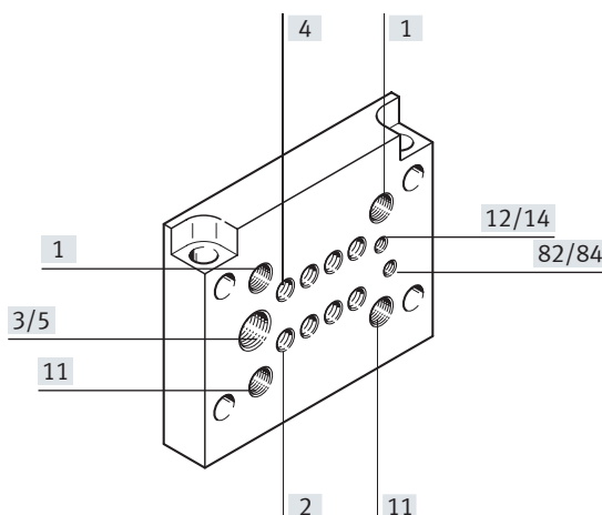
Pneumatischer Multipol
