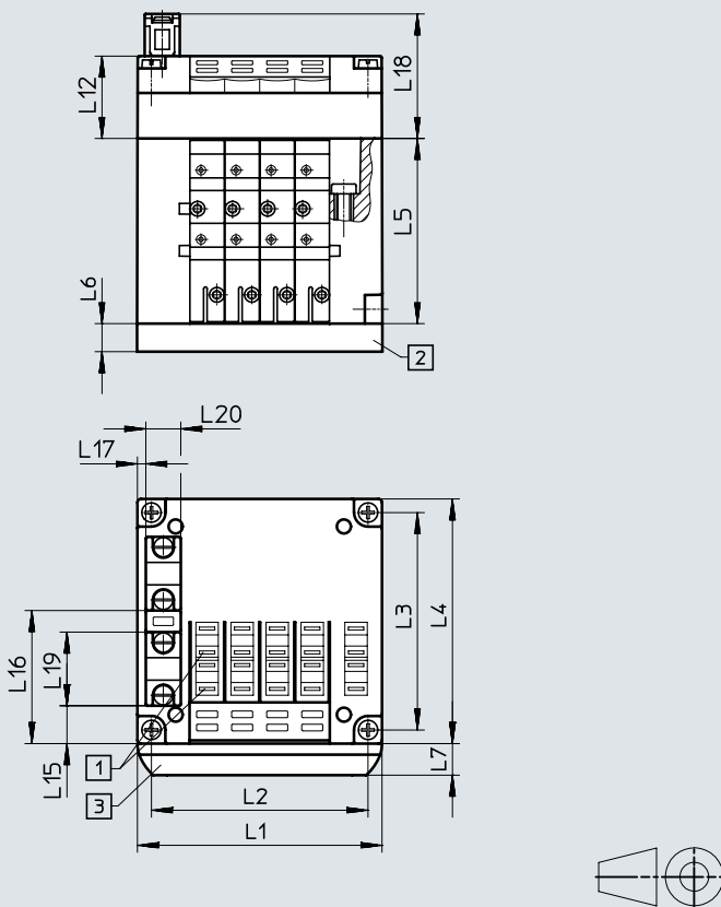
Ventilinsel mit AS-Interface-Anschluss – CPV10/14/18
