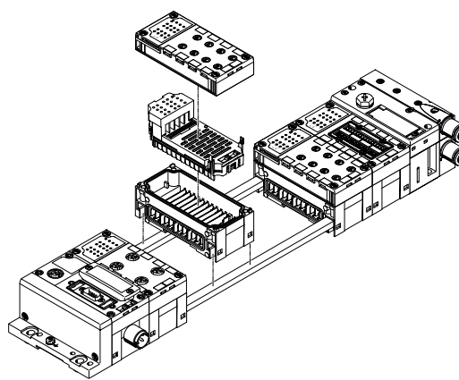
Modularität bei elektrischer Peripherie CPX
