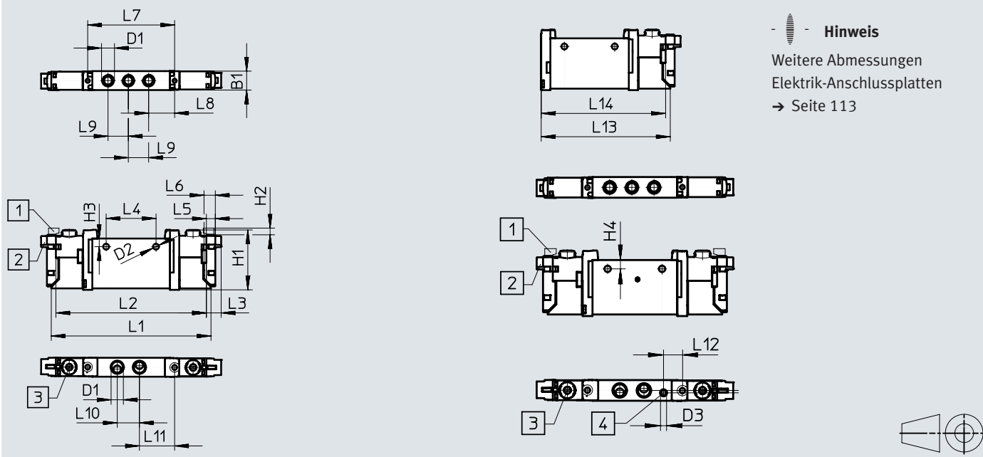
[1] Elektrischer Anschluss vertikal
