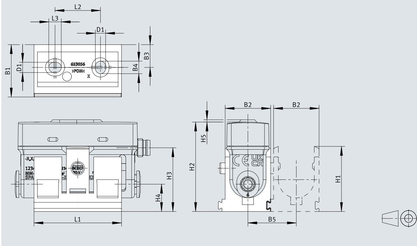
Dimensions – SPAF-...-MC-...
