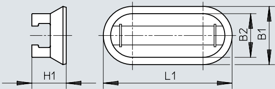
Dimensiones – Kit de fijación CRSMB
