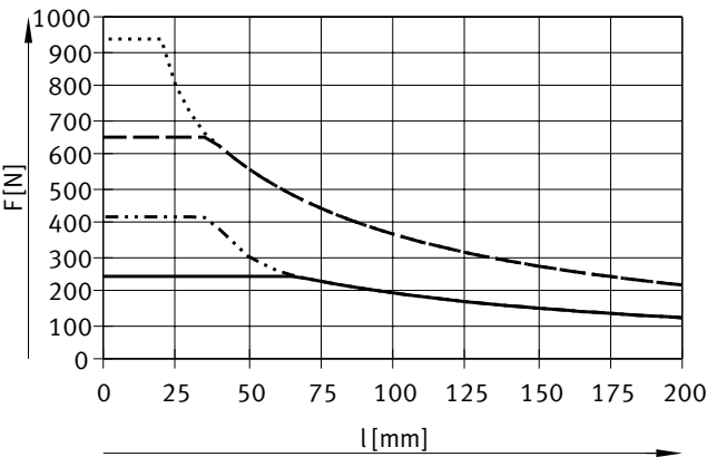
DFM-32 ... 63-KF, carrera de 80 ... 100 mm
