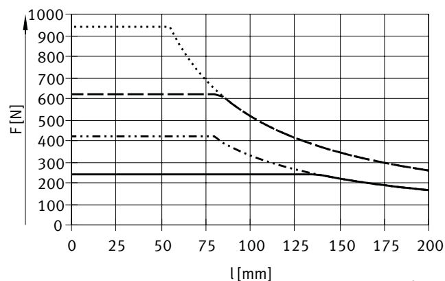
DFM-32 ... 63-GF, carrera de 125 ... 200 mm
