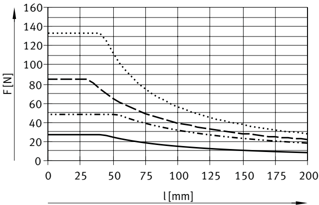
DFM-12 ... 25-KF, carrera de 30 mm
