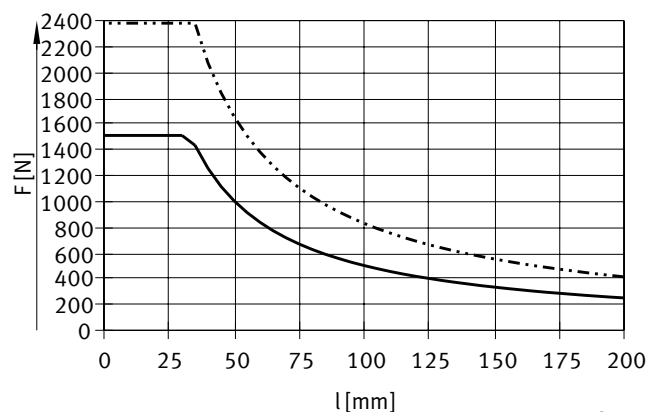
DFM-80 ... 100-GF, carrera de 25 mm
