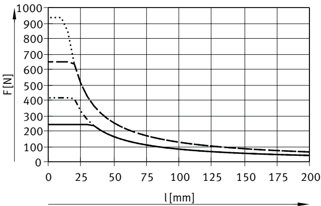
DFM-32 ... 63-KF, carrera de 50 mm
