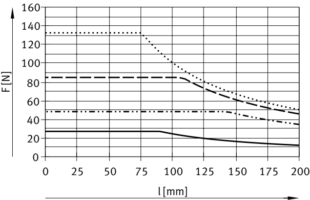
DFM-12 ... 25-KF, carrera de 40 ... 100 mm
