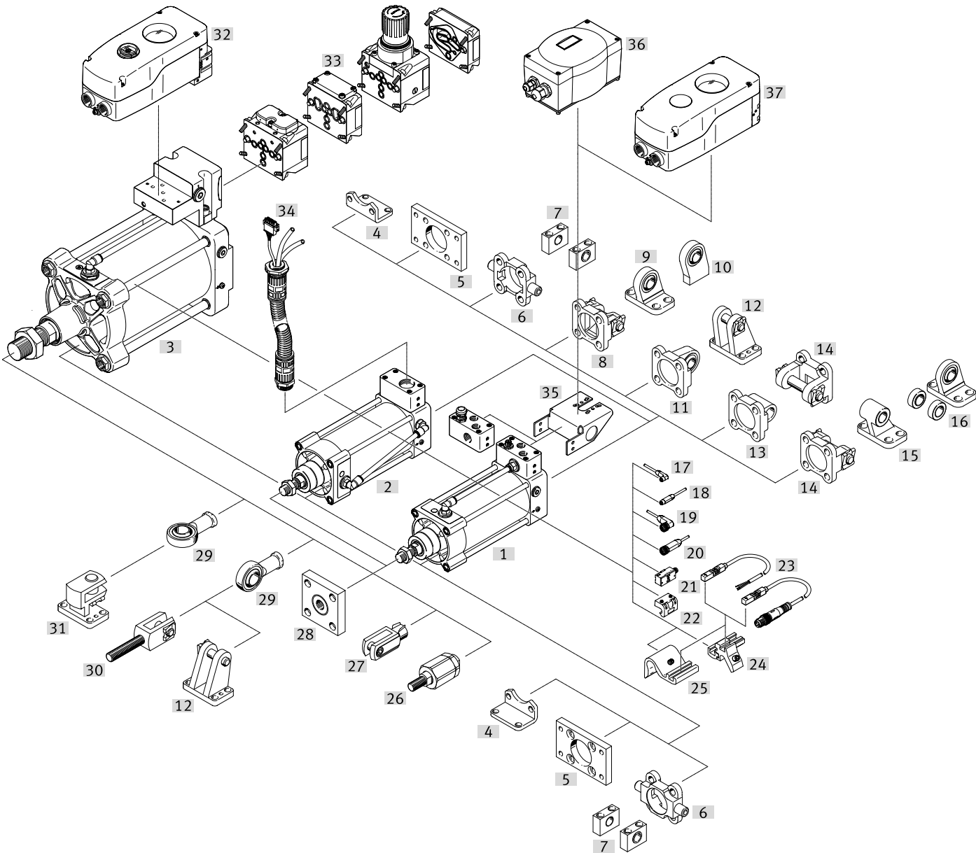
Cuadro general de periféricos ISO15552
