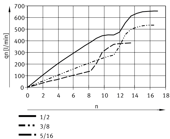
Caudal normal q_N con 6 \rightarrow 0 bar en función de las revoluciones del husillo n (GR-QB-1/2-U, GR-QB-3/8-U, GR-QB-5/16-U)
