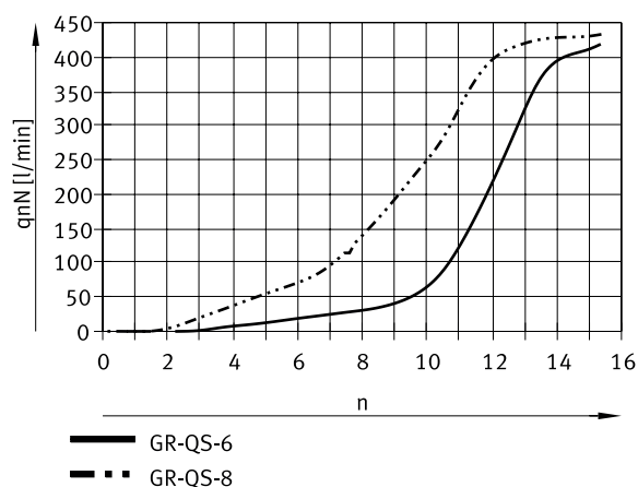
Caudal normal q_N con 6 \rightarrow 0 bar en función de las revoluciones del husillo n (GR-QS-6; GR-QS-8)
