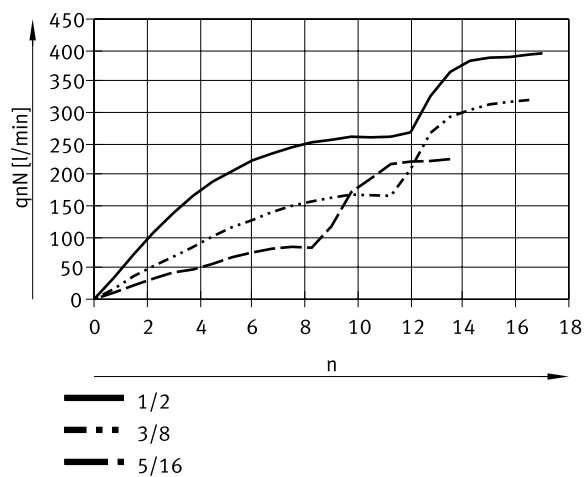
Caudal nominal normal q_N con 6 \rightarrow 5 bar en función de las revoluciones del husillo n (GR-QB-1/2-U, GR-QB-3/8-U, GR-QB-5/16-U)
