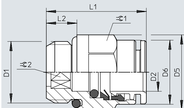
Dimensiones – Racor NPQH-D, rosca exterior, con hexágono exterior
