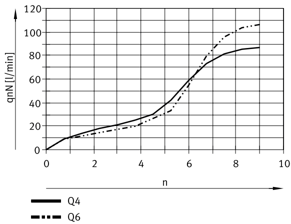
Caudal nominal normal q_{nN} a 0,6 \rightarrow 0,5 MPa en función de las revoluciones del husillo n para unión roscada M5, M7 (aire de entrada)
