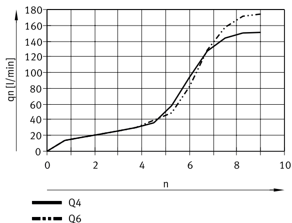
Caudal normal q_n a 0,6 \rightarrow 0 MPa en función de las revoluciones del husillo n para la unión roscada M5 (aire de escape)
