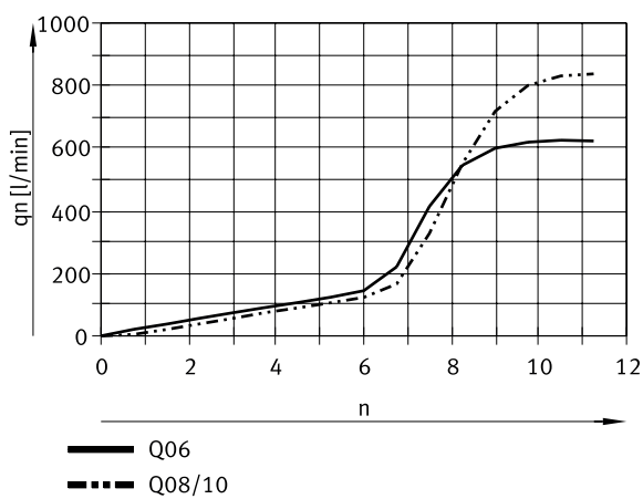
Caudal normal q_n a 0,6 \rightarrow 0 MPa en función de las revoluciones del husillo n para la unión roscada G1/4, R1/4 (aire de escape)
