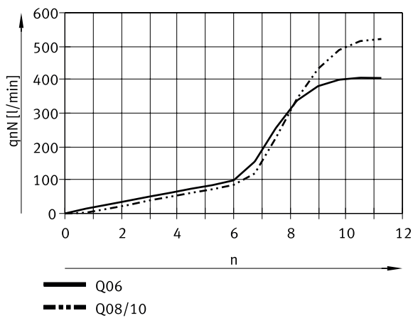
Caudal nominal normal q_{nN} a 0,6 \rightarrow 0,5 MPa en función de las revoluciones del husillo n para la unión roscada G1/4, R1/4 (aire de escape)
