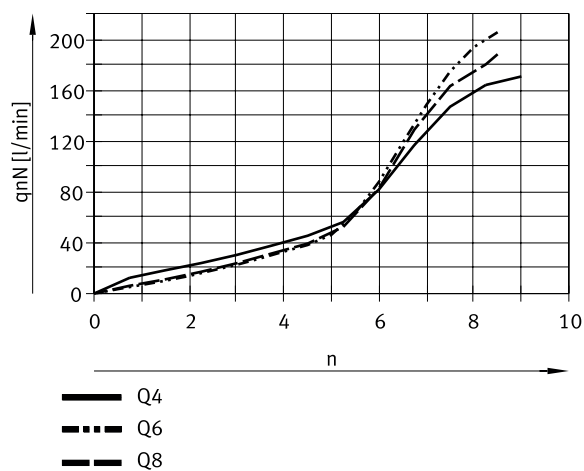
Caudal nominal normal q_{nN} a 0,6 \rightarrow 0,5 MPa en función de las revoluciones del husillo n para la unión roscada G1/8, R1/8 (aire de escape)
