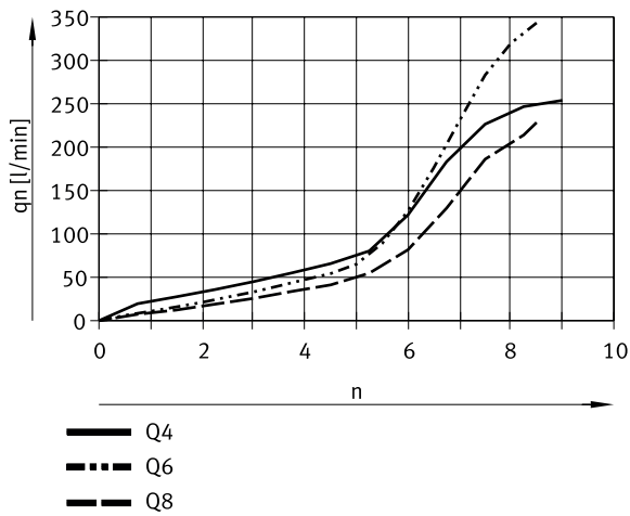
Caudal normal q_n a 0,6 \rightarrow 0 MPa en función de las revoluciones del husillo n para la unión roscada G1/8, R1/8 (aire de escape)
