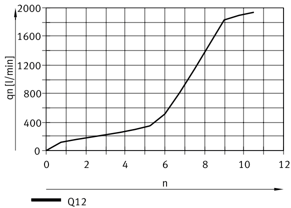
Caudal normal q_n a 0,6 \rightarrow 0 MPa en función de las revoluciones del husillo n para la unión roscada G1/2, R1/2 (aire de escape)
