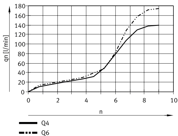
Caudal normal q_n a 0,6 \rightarrow 0 MPa en función de las revoluciones del husillo n para unión roscada M5, M7 (aire de entrada)
