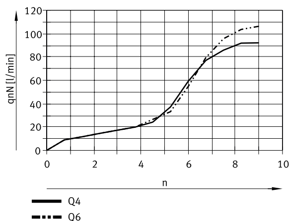
Caudal nominal normal q_{nN} a 0,6 \rightarrow 0,5 MPa en función de las revoluciones del husillo n para la unión roscada M5 (aire de escape)
