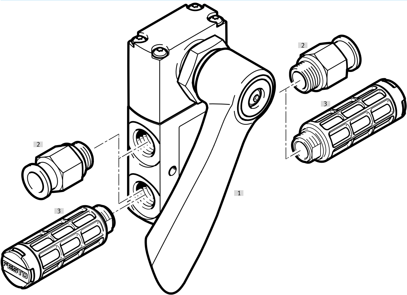
Cuadro general de periféricos para válvula de palanca manual, lateral, accionamiento manual 3/2
