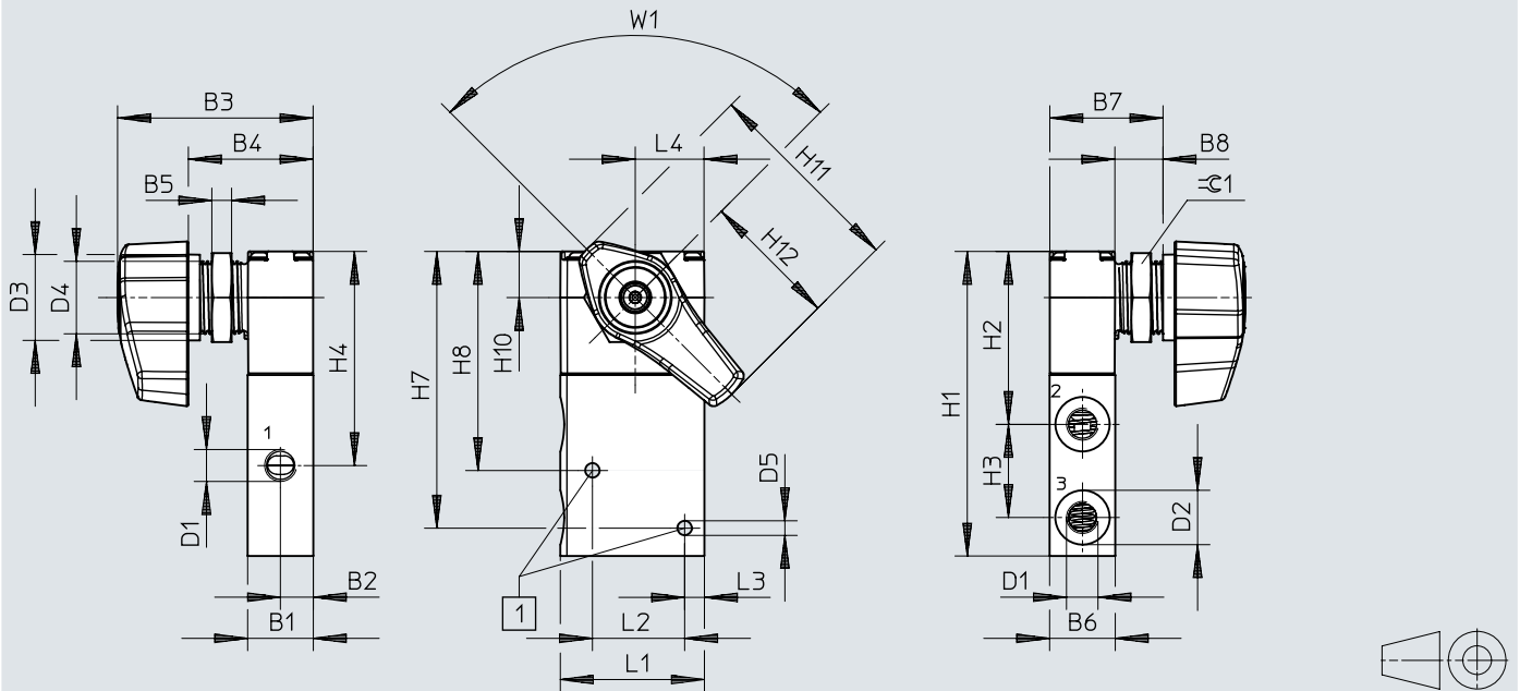
Dimensiones – Válvula de 3/2 vías, válvula selectora, lateral
