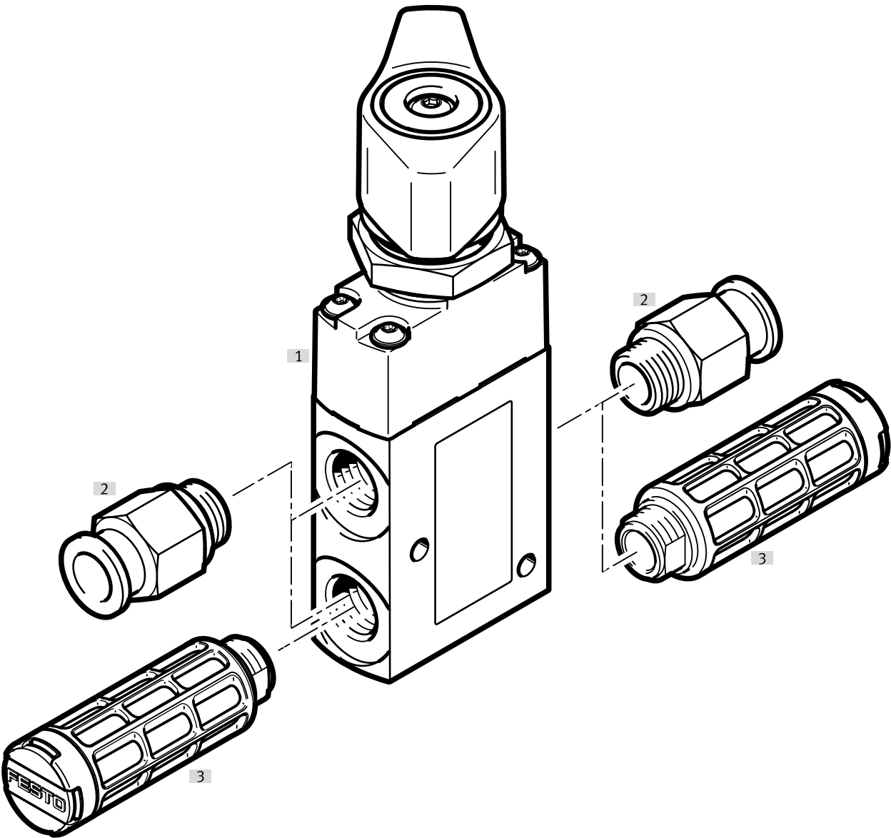
Cuadro general de periféricos para válvula selectora, accionamiento manual 3/2
