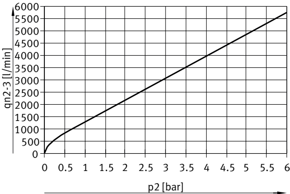
Caudal qn de 2 -> 3 en función de la sobrepresión de salida p2, VPPM-12L-...-0L6H-... (8 bar)
