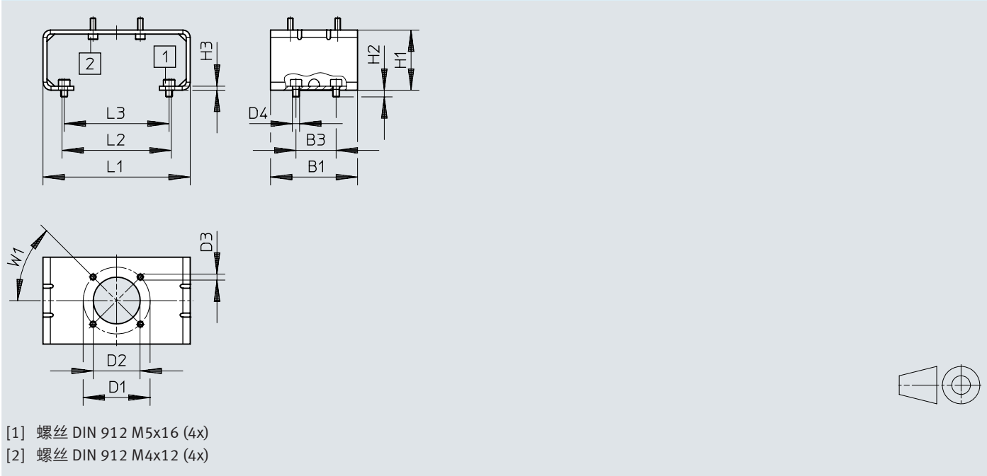
尺寸 – 安装转接件 DARQ-K-P-...
