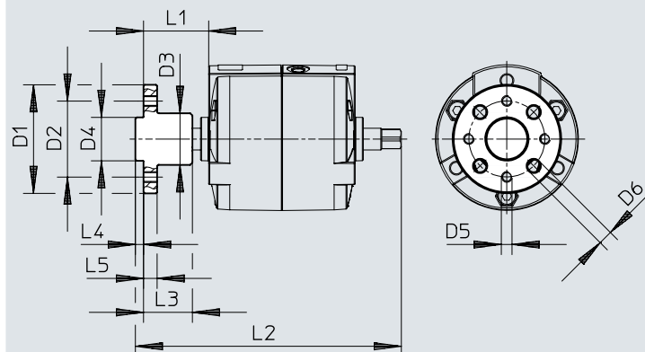
尺寸 – 嵌入式法兰 DARF-Q12-12 ... 16
