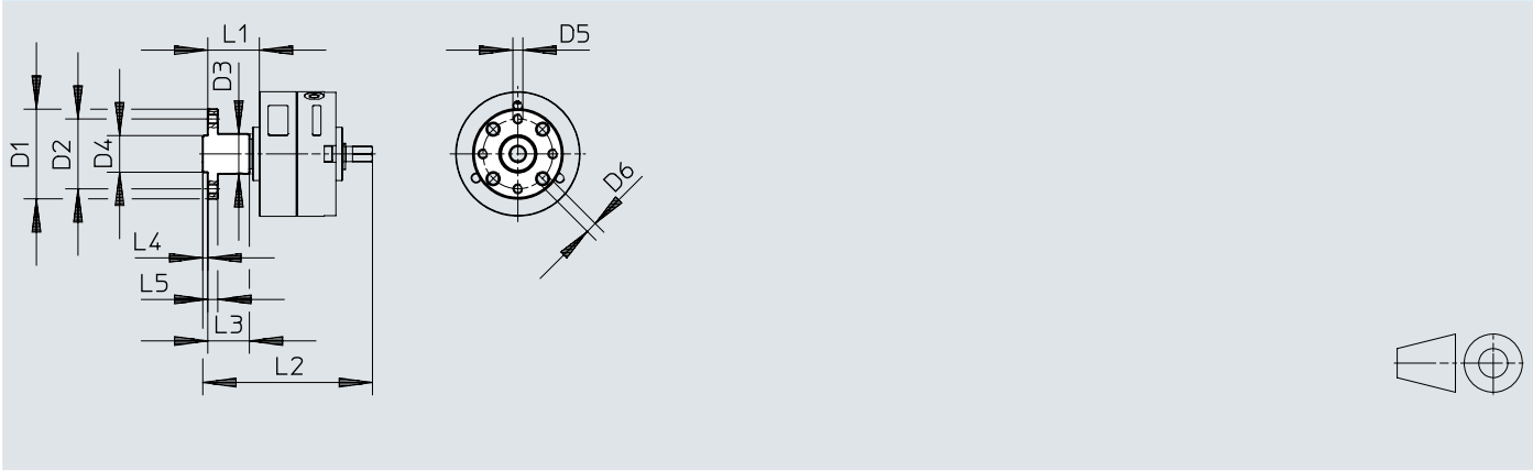
尺寸 – 嵌入式法兰 FWSR
