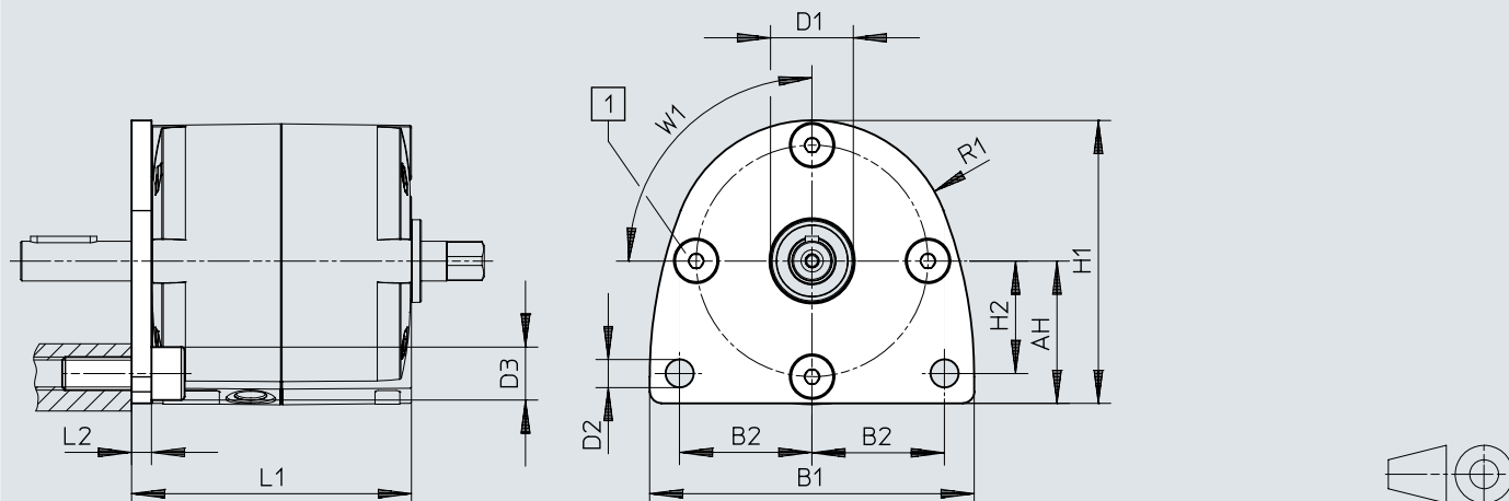
尺寸 – 法兰安装件 DAMF-Q12-32 ... 40
