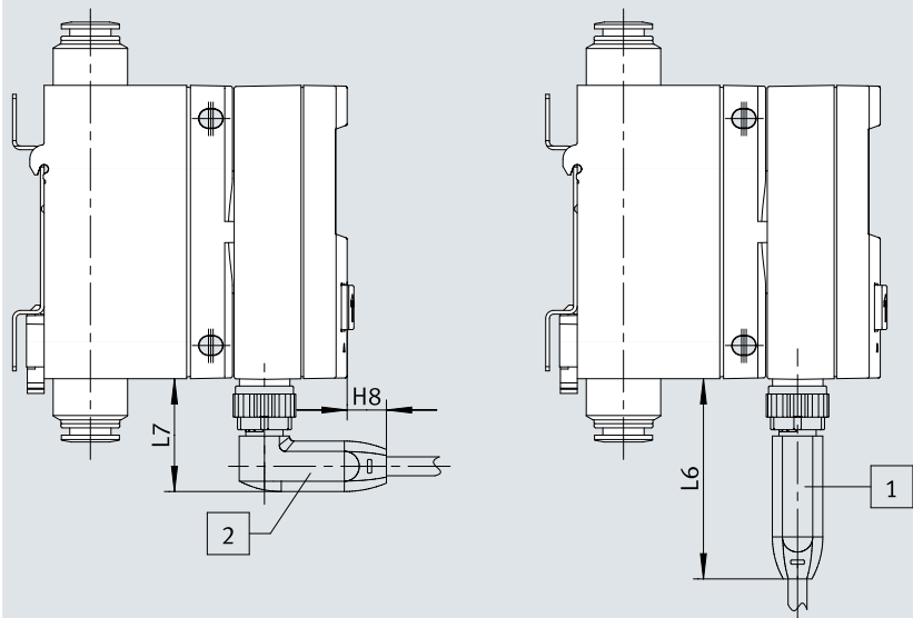
尺寸 – SFAB-...-PNLK-...
