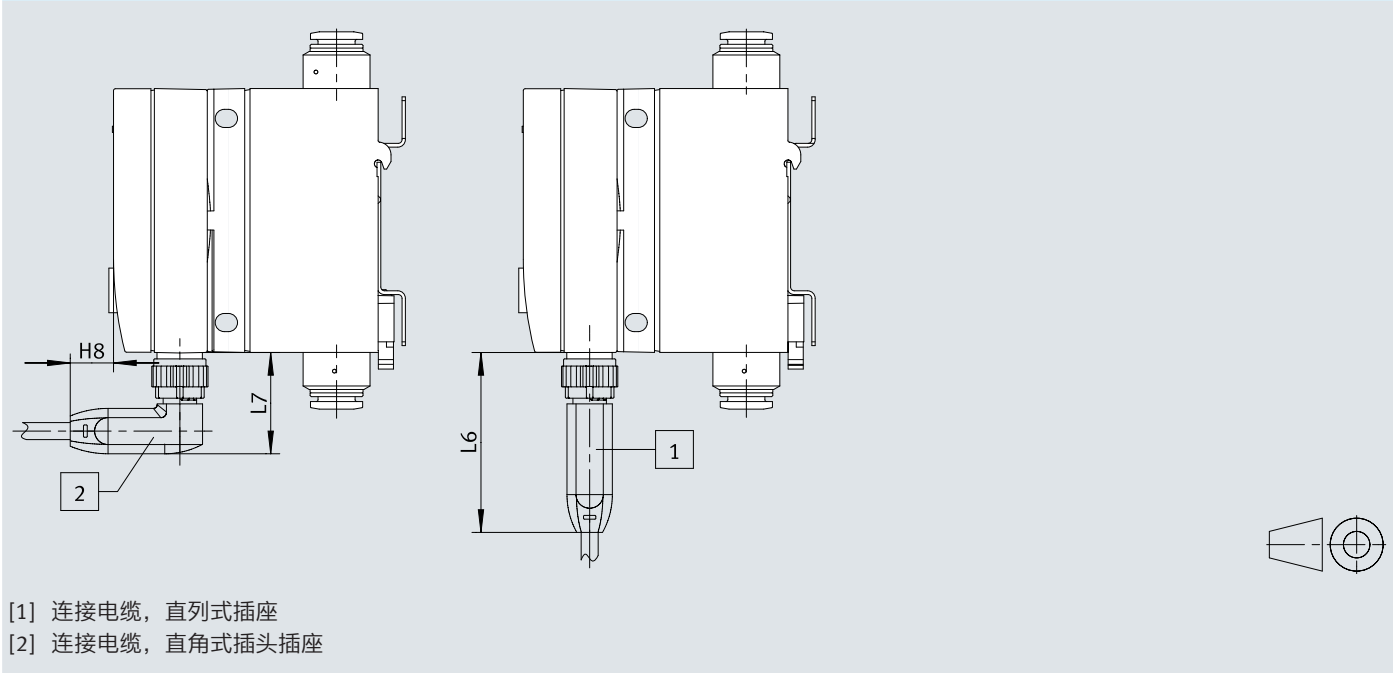
尺寸 – SFAB-...-2SA/2SV-...
