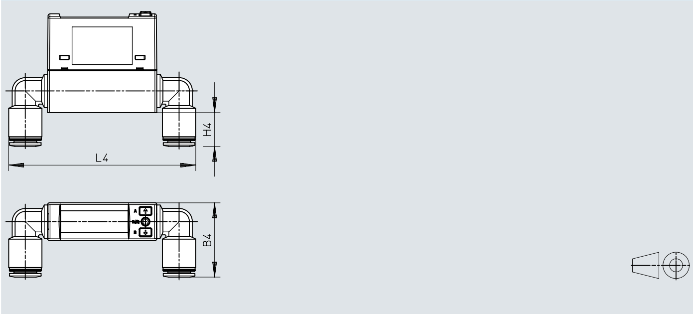
尺寸 – SFAH-...-Q...AR-...
