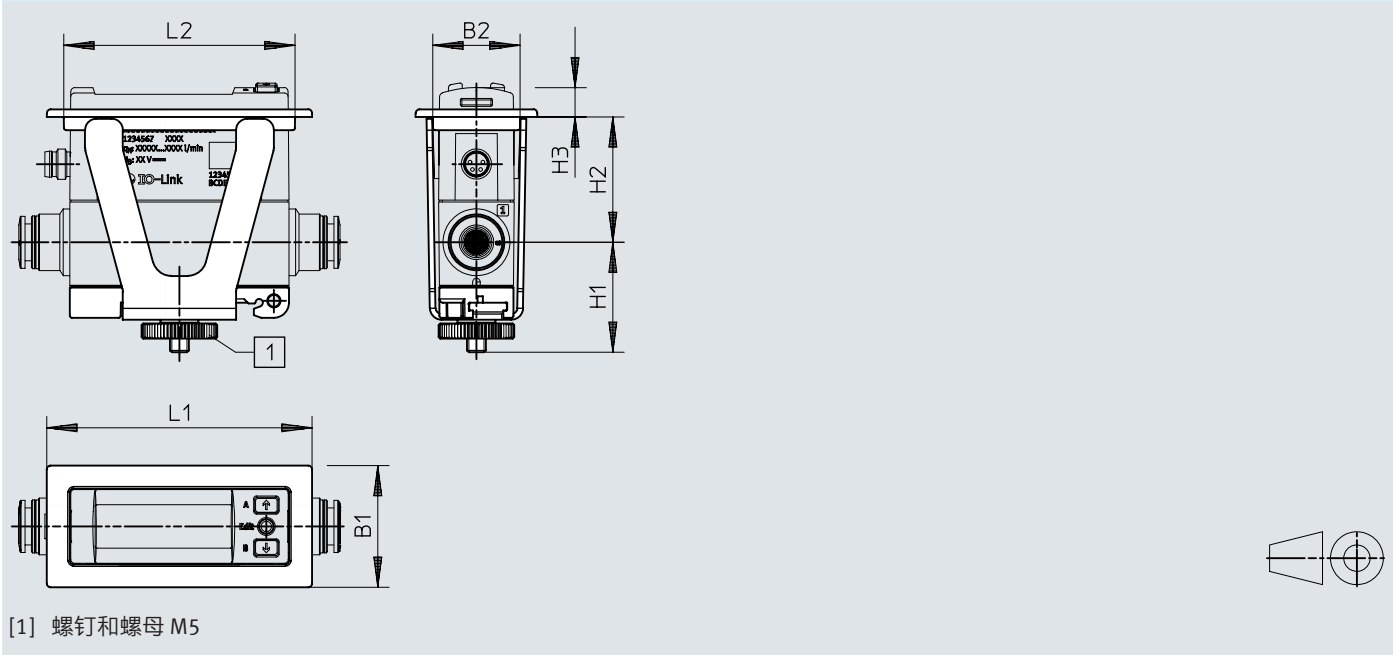
尺寸 – 面板式安装组件 SAMH-FH-F
