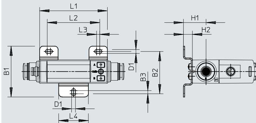
尺寸 – 墙面安装元件 SAMH-FH-W
