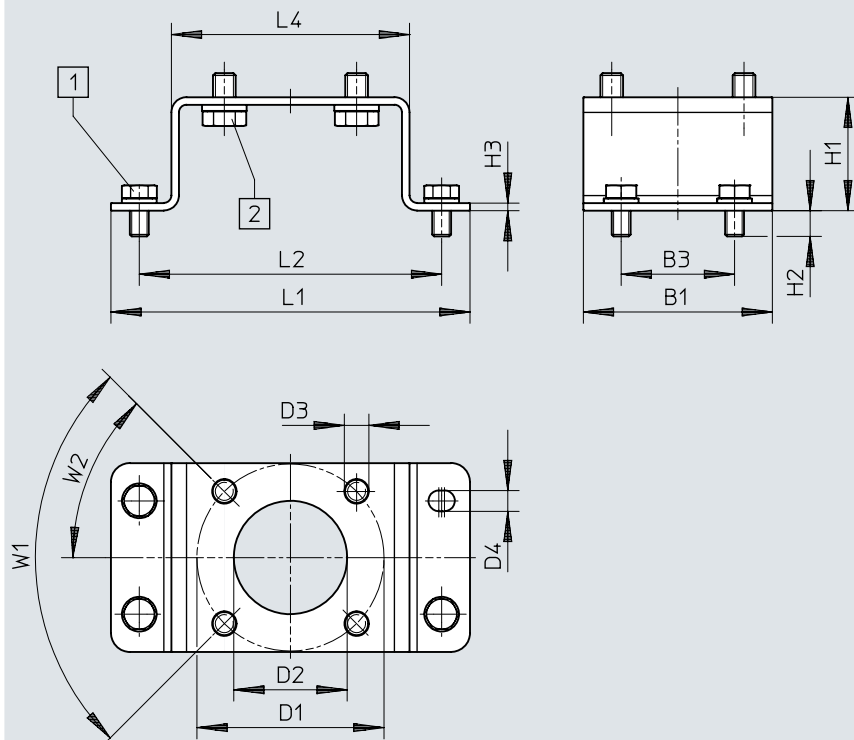
尺寸 – 安装转接件 DARQ-K-X1-A1-F05-...-R1
