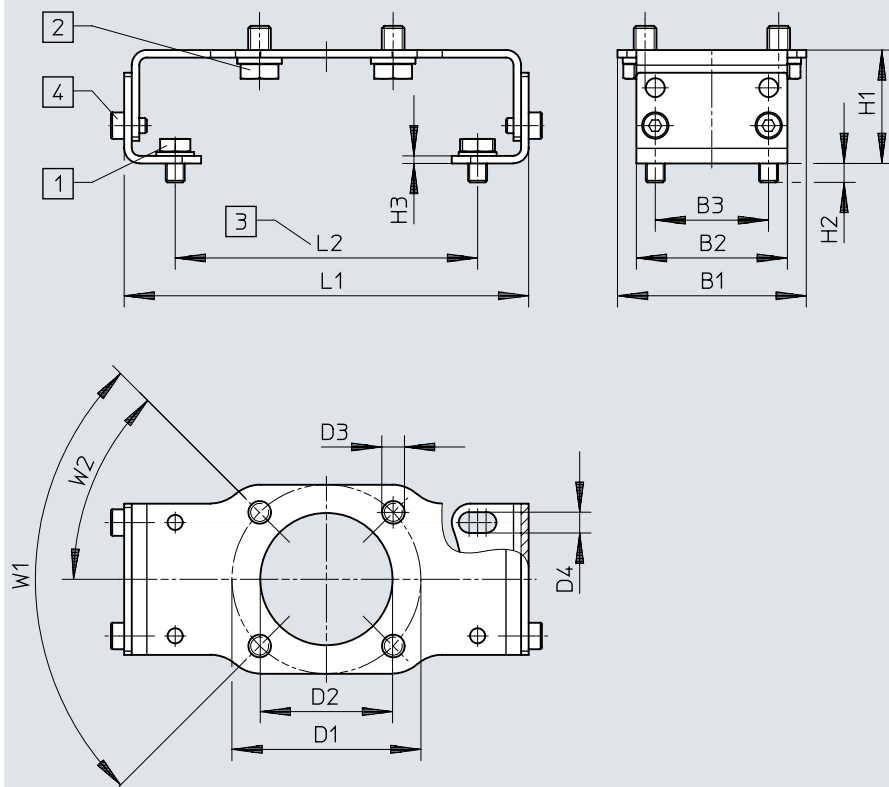
尺寸 – 安装转接件 DARQ-K-X1-A3-F05-20-R1
