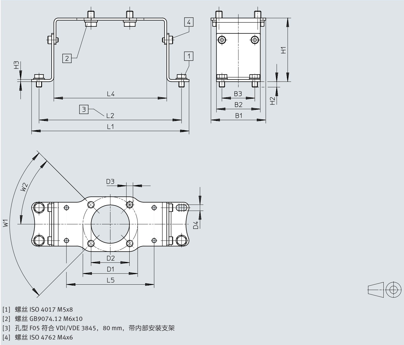
尺寸 – 安装转接件 DARQ-K-X1-A3-F05-50-R1
