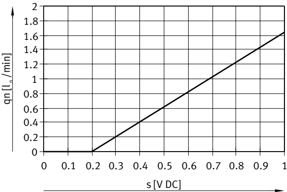
流量 q_n 与设定值 s 的关系，详细范围，公称口径 1.4 mm
