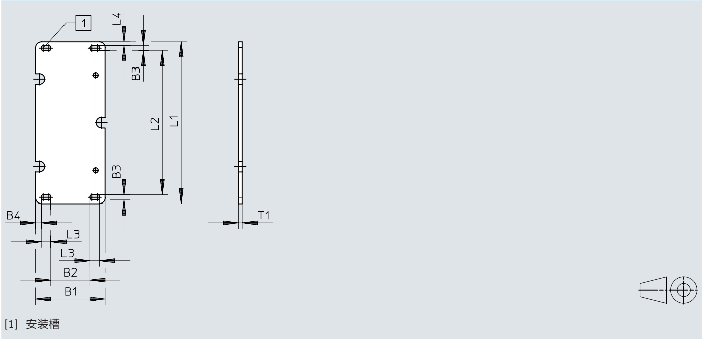
尺寸 – 墙面安装组件 VAME-P14-W
