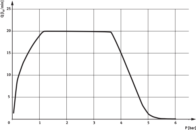
室温下，最大流量与工作压力关系示意图，公称口径 1.4 mm
