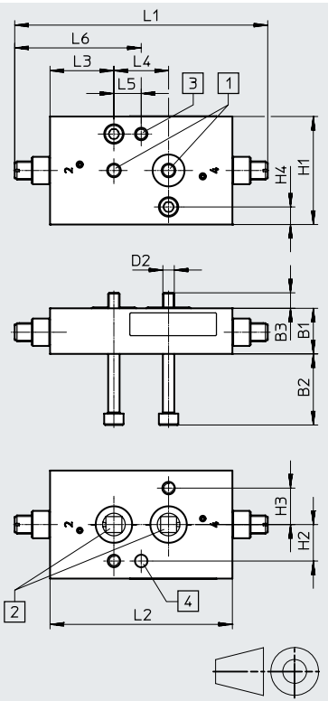
双作用 VABF-...P2
