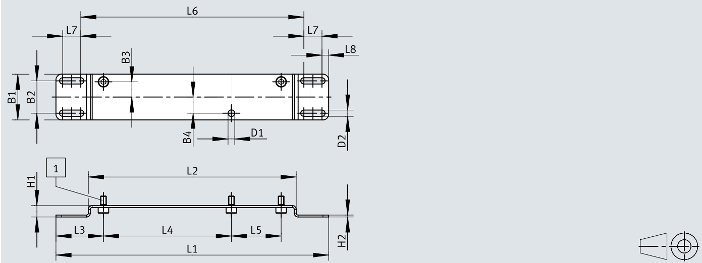
[1] Schraube M3x6
