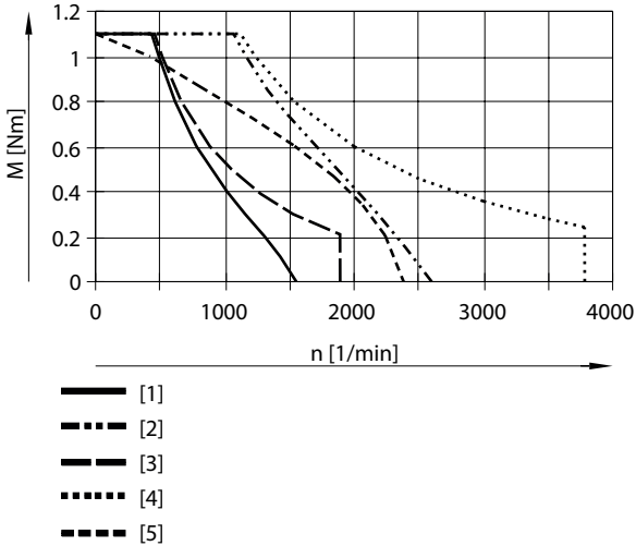
用于 EMMT-ST-57-M 时扭矩 M 与转速 n 的关系
