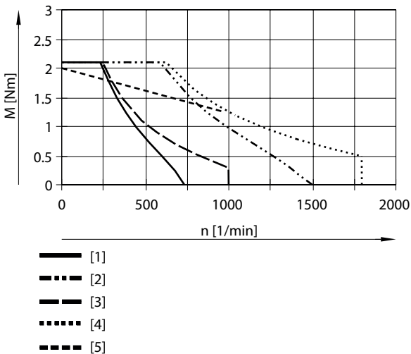
用于 EMMT-ST-57-L 时扭矩 M 与转速 n 的关系
