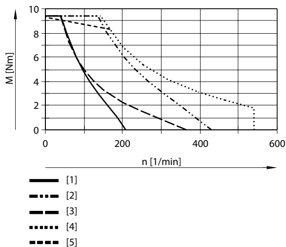
用于 EMMT-ST-87-L 时扭矩 M 与转速 n 的关系
