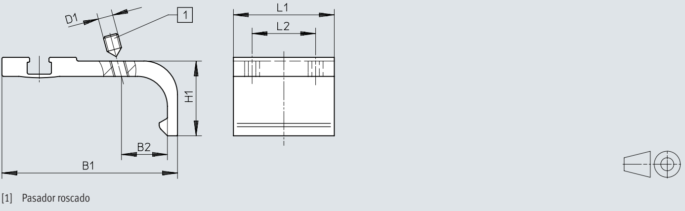
Dimensiones – Kit de fijación SMB-8-FENG
