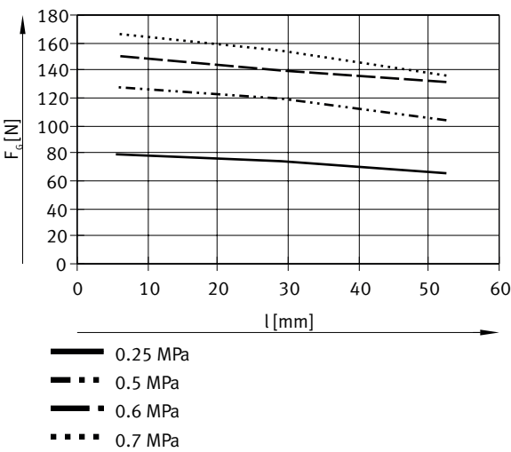
每个抓手指的抓取力 FGr 与气源压力和杠杆臂 x 的关系 – 外部抓取（合拢），双作用
