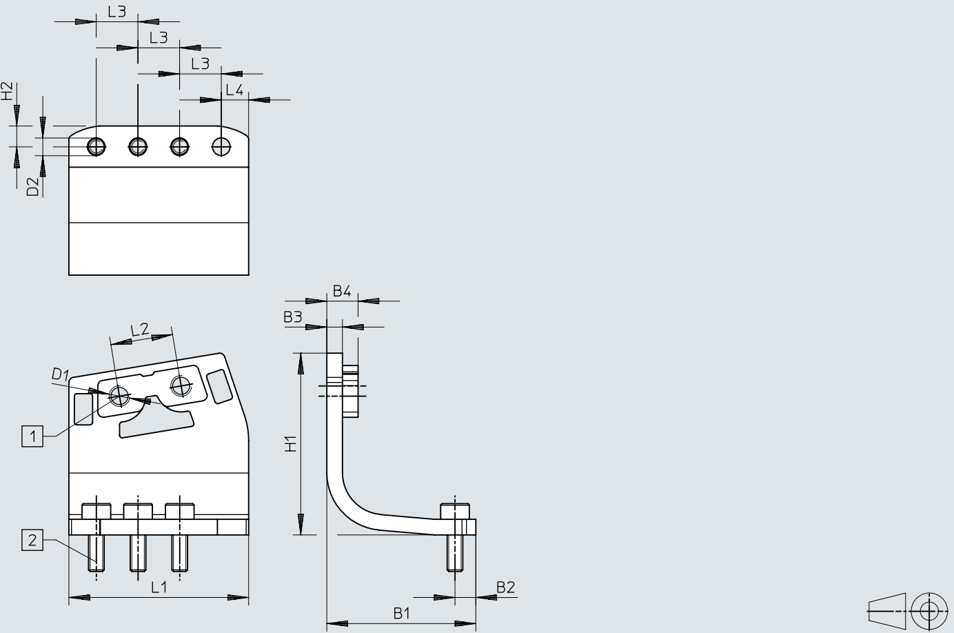
尺寸 – 安装支架 DHAS-MA-B6-80
