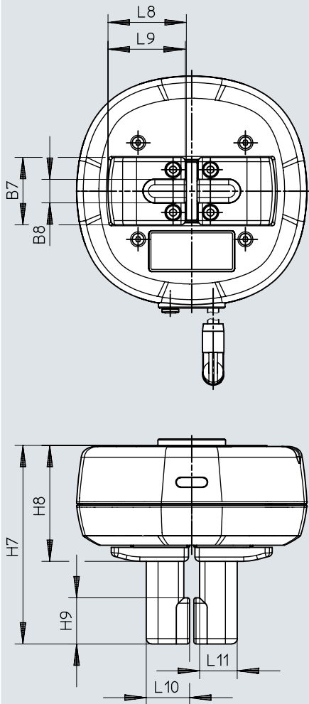
尺寸 – 平行抓手 HPPH, 带抓手手指 HAFH-B30-16-45-N
