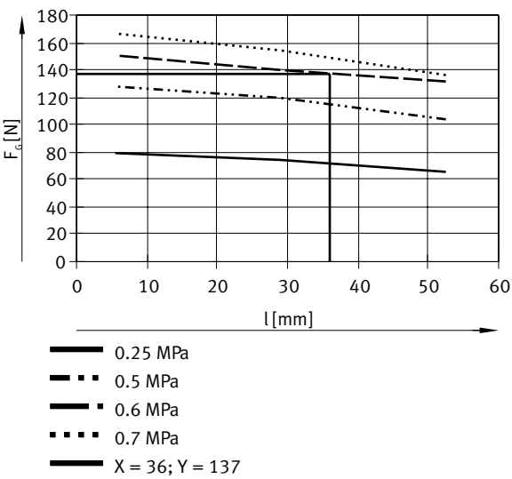
每个抓手手指的抓取力 F_{Gr} ，在 0.6 MPa（6 bar，87 psi）时，与杠杆臂 x 及偏心率 a 和 b 的关系
