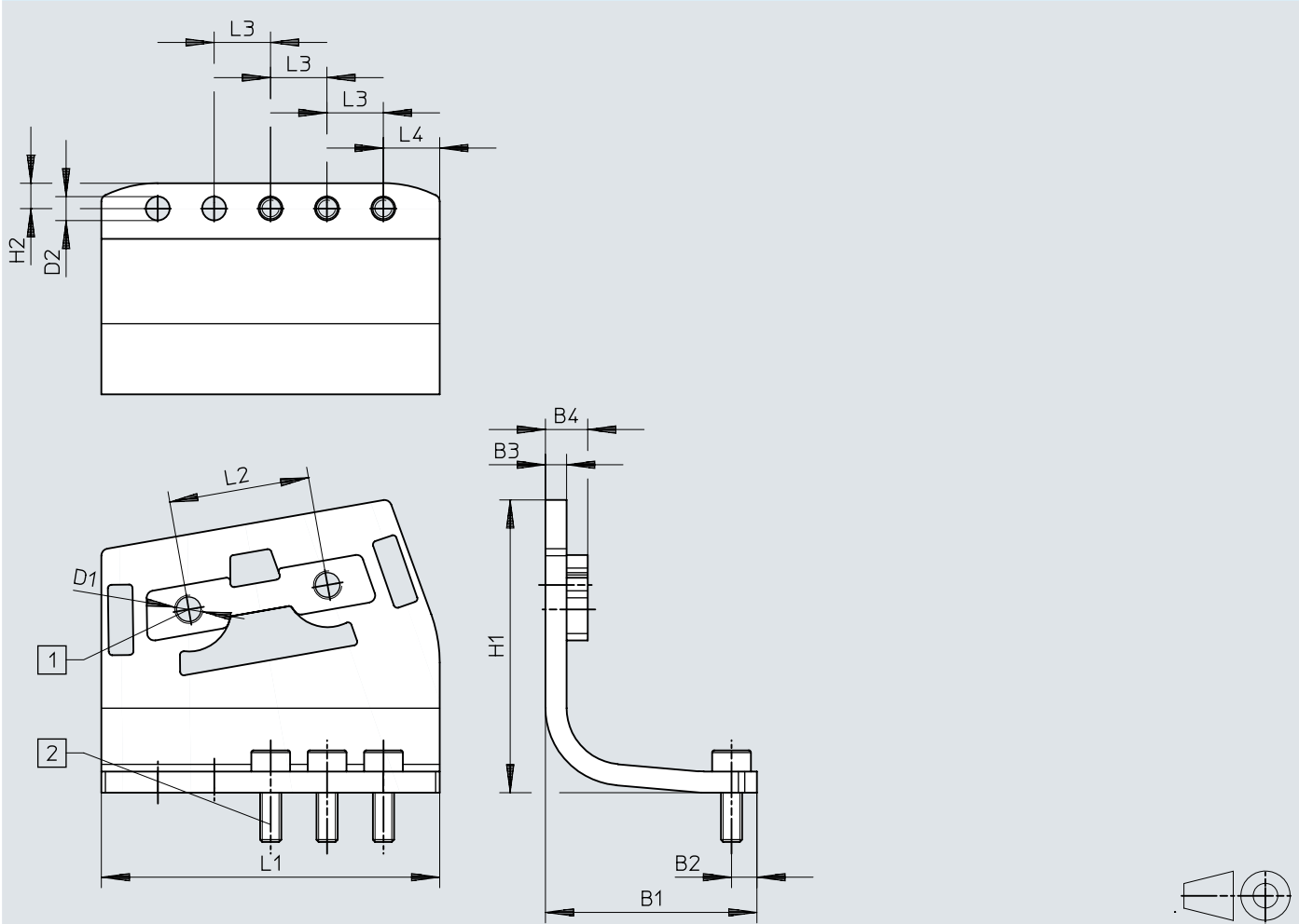
尺寸 – 安装支架 DHAS-MA-B6-120
