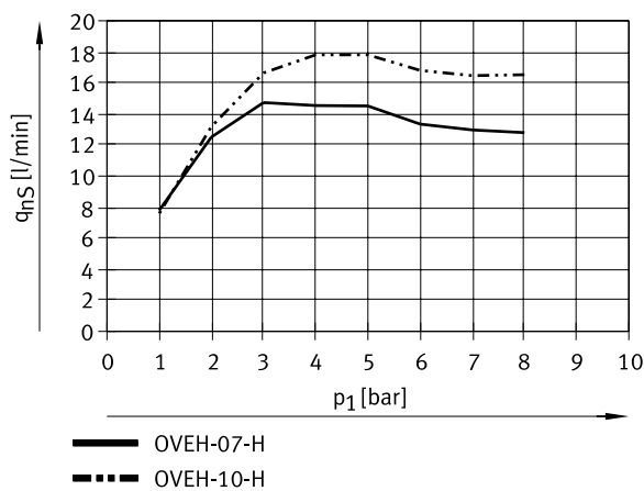
Saugvolumenstrom q_{nS} gegen Atmosphäre in Abhängigkeit Betriebsdruck p_1 (Hohes Vakuum)
