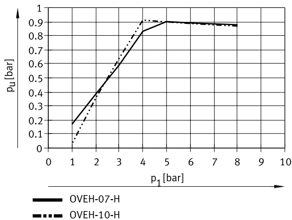
Vakuum p_U in Abhängigkeit vom Betriebsdruck p_1 (Hohes Vakuum)
