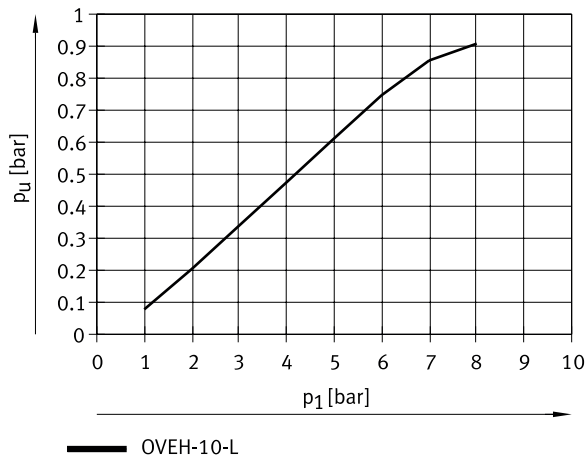
Vakuum p_U in Abhängigkeit vom Betriebsdruck p_1 (Hoher Saugvolumenstrom)
