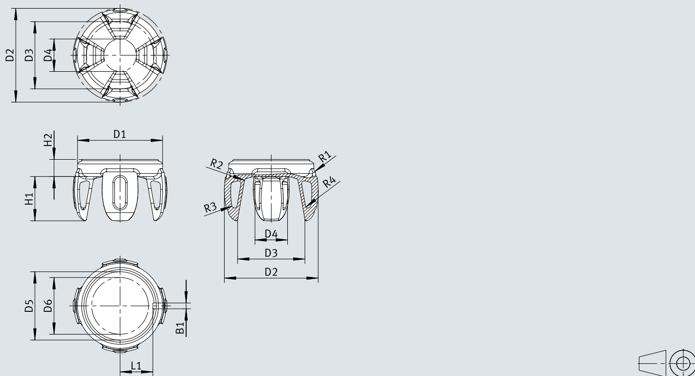
Dimensiones – Tapa para dedos de sujeción HAMA-GA-B33-70-4-S-40-BU
