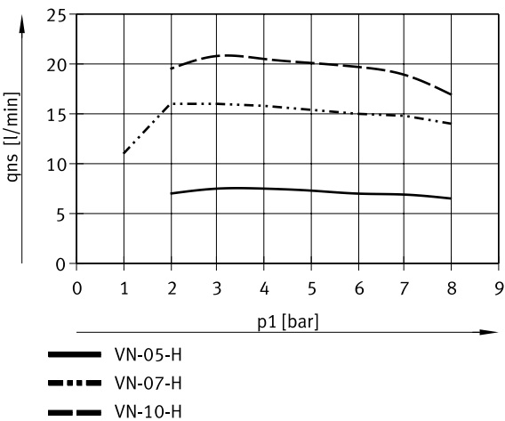
Caudal de aspiración q_{ns} (contra atmósfera) en función de la presión de funcionamiento p_1 - Alto vacío (estándar; VN-05/07/10)
