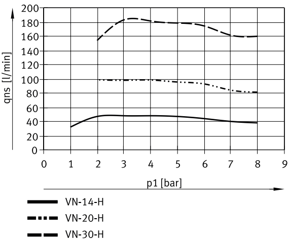
Caudal de aspiración q_{ns} (contra atmósfera) en función de la presión de funcionamiento p_1 - Alto vacío (estándar; VN-14/20/30)
