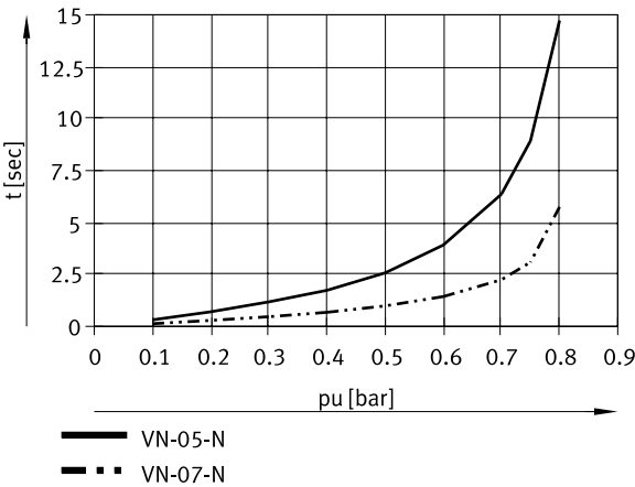
Tiempo de evacuación t en función del vacío p_u para un volumen de 1 l con una presión de funcionamiento de 6 bar – Alto caudal de aspiración (Inline; VN-05/07)
