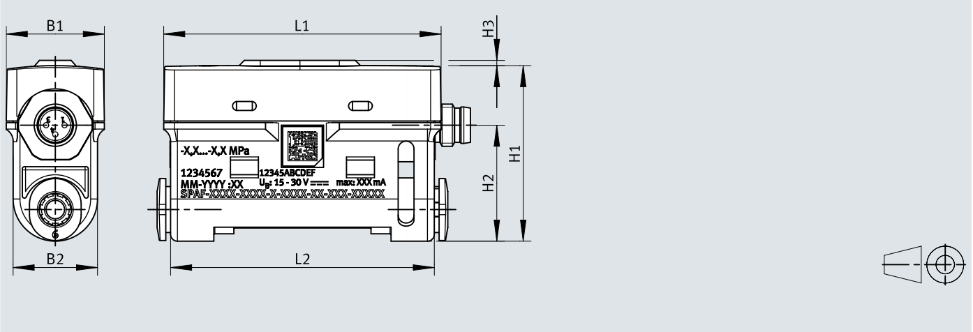
尺寸 - SPAF-...
