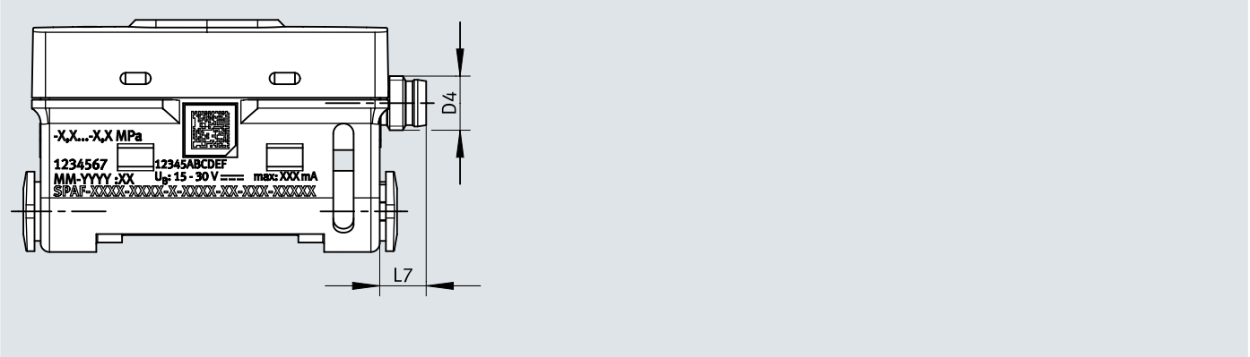
尺寸 - SPAF-...-M8-...
