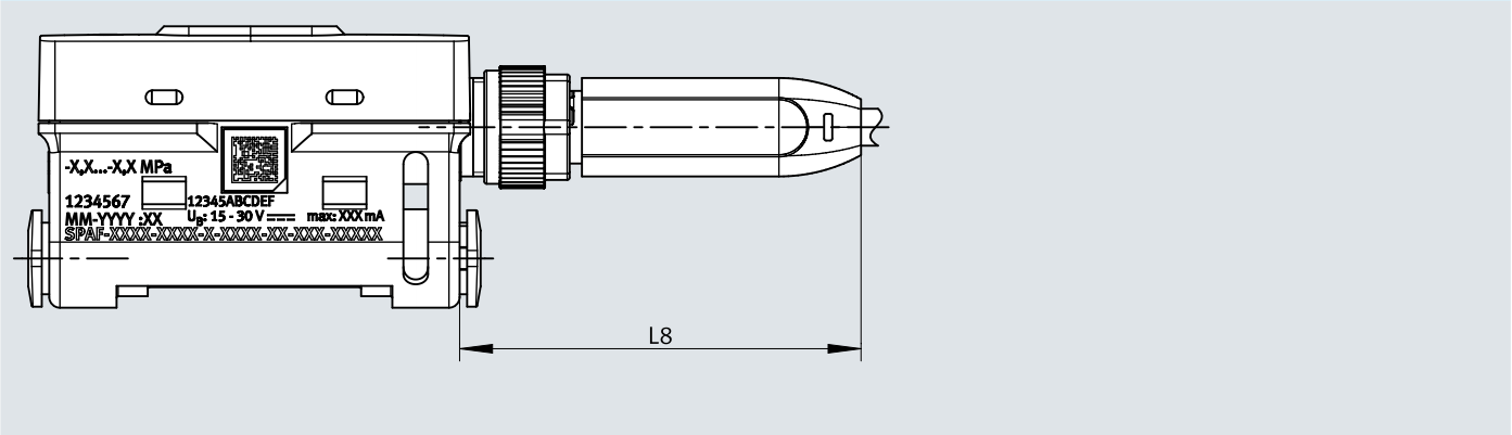
尺寸 - SPAF-...-M12-...S
