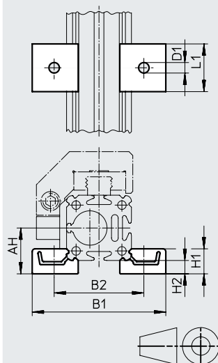
Kolben-Ø 18 und 25
