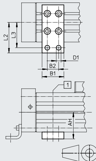
Kolben-Ø 32 ... 63
