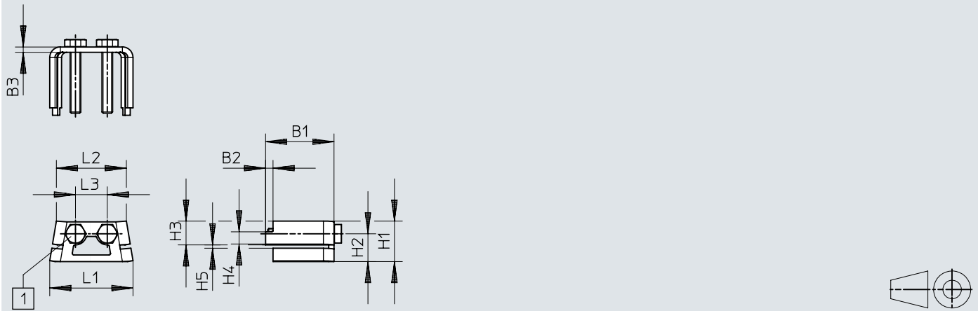
寸法 – 取付キット DHAS-ME-H9-60/80
