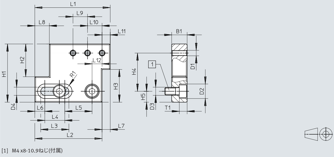
寸法 - 中間プレート HAMF-PA
