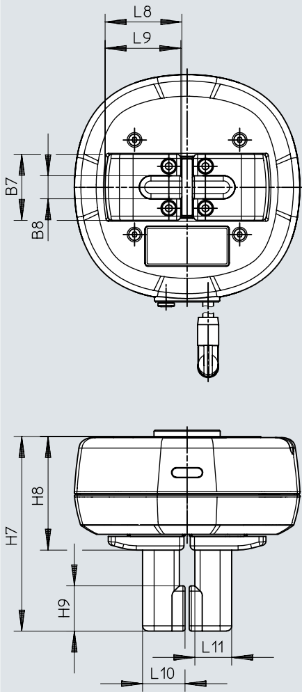
寸法 – パラレルグリッパ HPPH, グリッパフィンガ付 HAFH-B30-16-45-N
