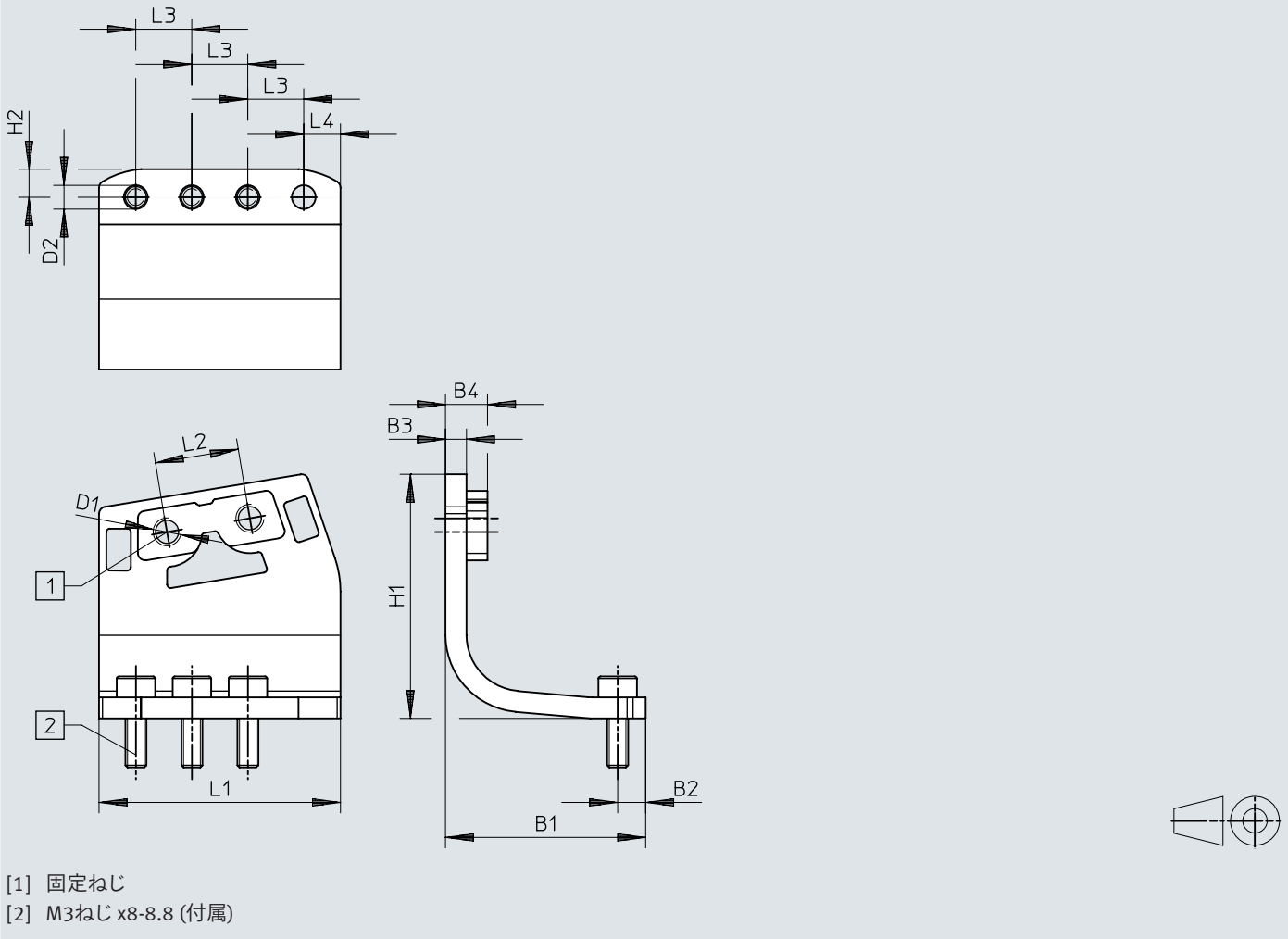
寸法 – 取付ブラケット DHAS-MA-B6-80
