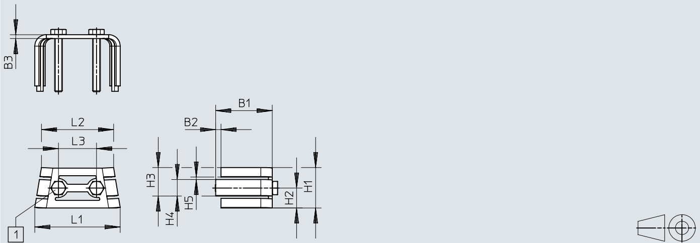
[1] DHAS-ME-H9-120:ねじ(ISO 4017-M4x30-A2-70, 付属)
