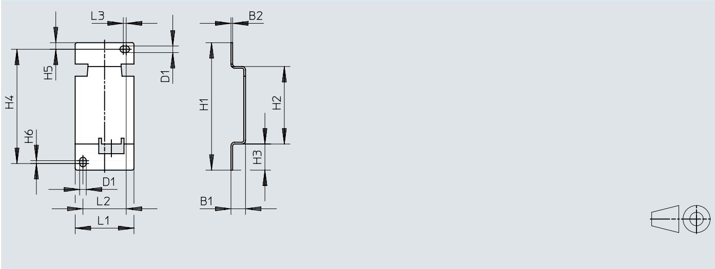
치수 - 어댑터 플레이트 SDE1- ...-W ...
