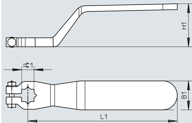
Kích thước – Cánh tay đòn VAOH, 3 chiều
