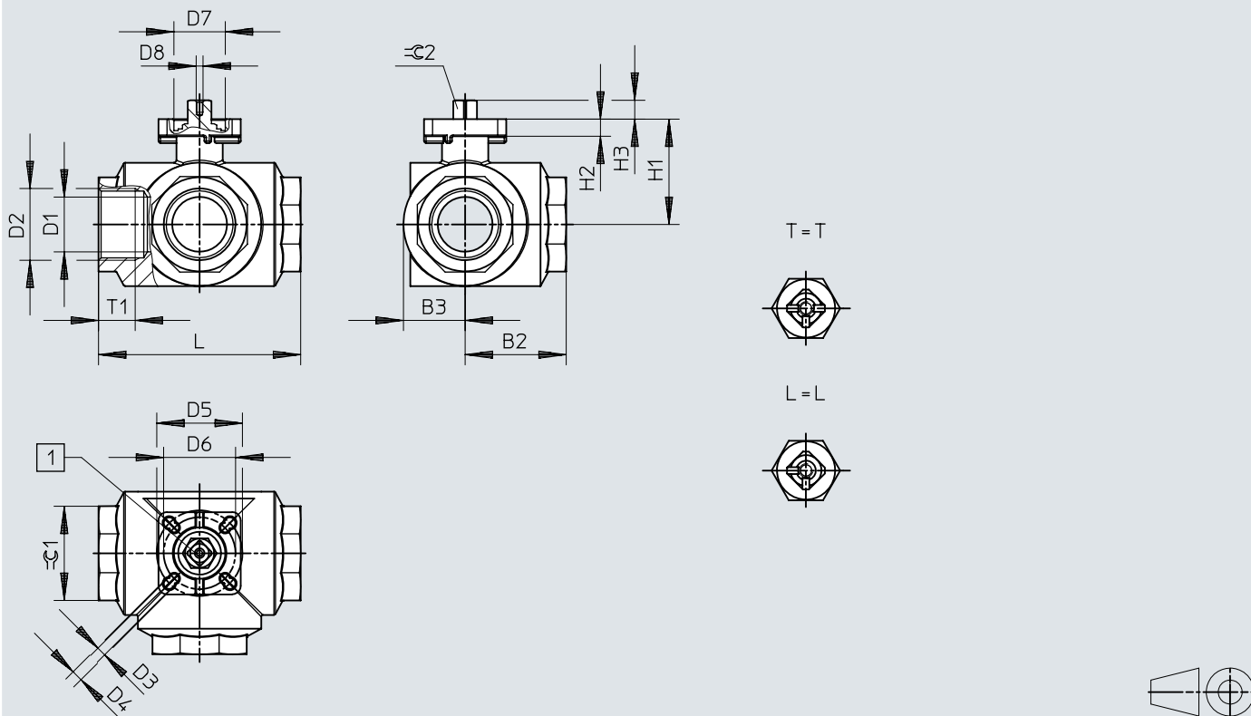
Kích thước – Van bi VZBM, 3 chiều
