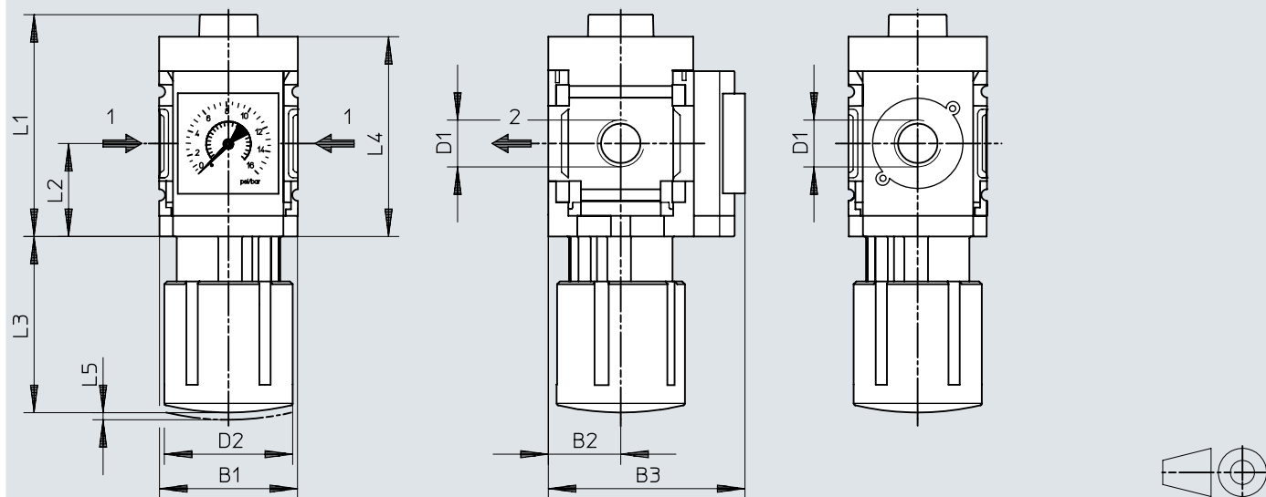
Dimensions – Position de montage alternative, bouton rotatif en bas
