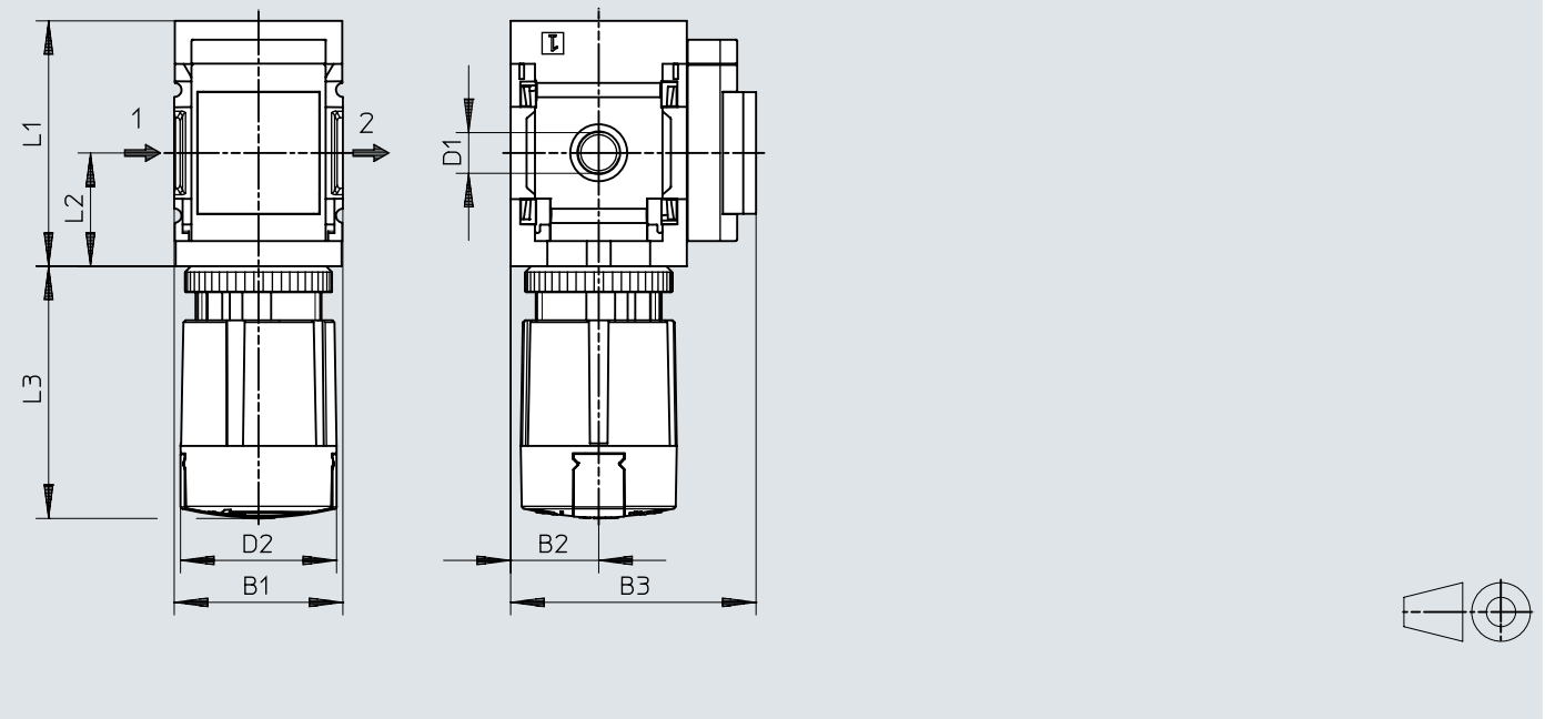
Dimensions – Position de montage alternative, bouton de réglage en bas
