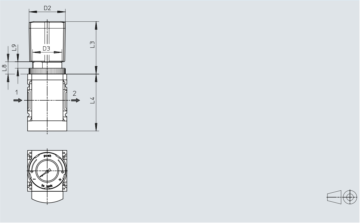
Dimensions – Manomètre à bouton de réglage, petit
