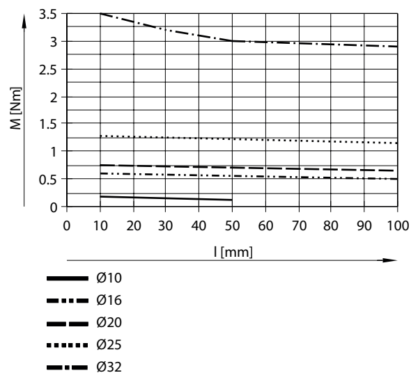
Dopušteni moment M ovisno o hodu L - prolazna klipnjača - Vodilica s kugličnim ležajem
