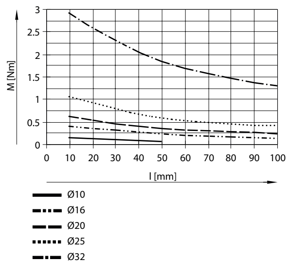
Dopušteni moment M ovisno o hodu L - Jednostrana klipnjača - Vodilica s kugličnim ležajem
