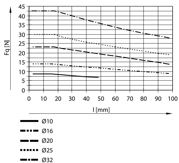
允許的橫向力 F 與行程 L 的關係 - 單側活塞桿 - 循環滾珠軸承導軌
