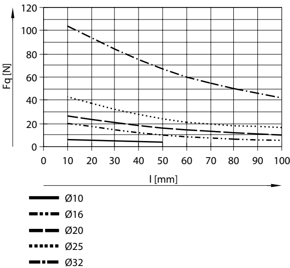
允許的橫向力 F 與行程 L 的關係 - 單側活塞桿 - 滑動導軌
