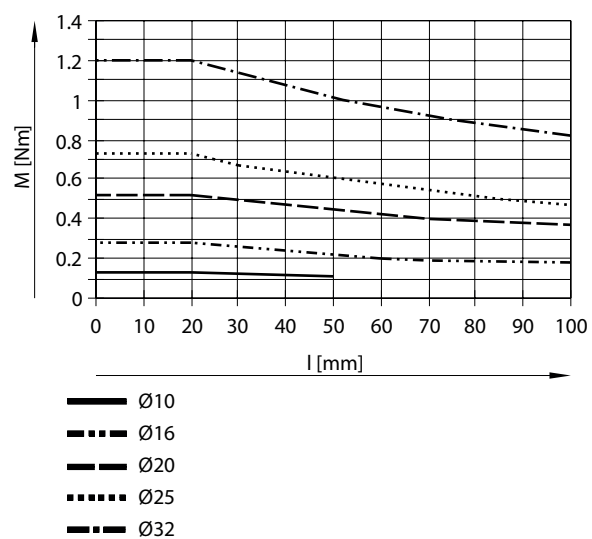
允許的扭矩 M 與行程 L 的關係 - 貫通活塞桿 - 循環滾珠軸承導軌
