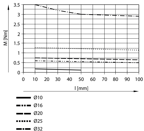
允許扭力 M 取決於行程 L - 通過活塞桿 - 滑動導軌
