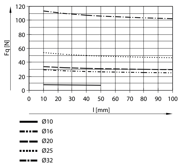
允許的橫向力 F 與行程 L 的關係 - 貫通活塞桿 - 滑動導軌
