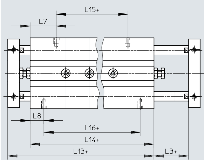
尺寸 – DPZJ-10/-16-...-S2 – 附雙端板和貫通活塞桿
