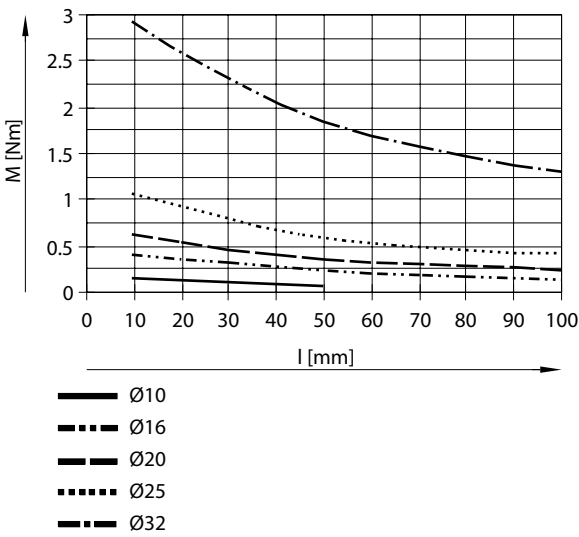
允許扭矩 M 取決於行程 L - 單側活塞桿 - 滑動導軌
