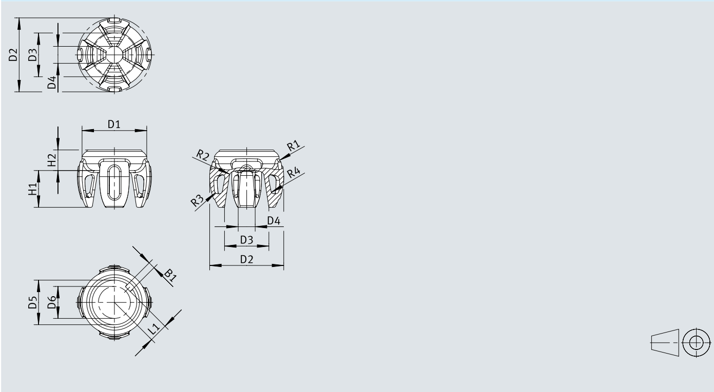
치수 - 그리퍼 핑거 캡 HAMA-GA-B33-40-4-S-40-BU
