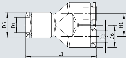
Méretetek – NPQM-YY-csatlakozó, szűkített
