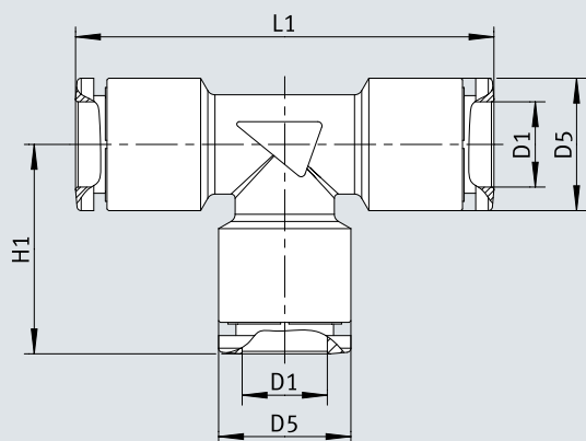
Méretetek – NPQM-T dugaszolható T-csatlakozó
