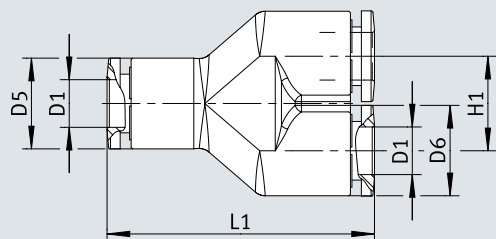
Méretek – NPQM-Y Y-csatlakozó
