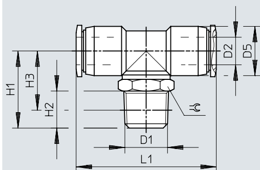
Dimensions – Raccord enfichable en T QBMT, filetage NPT
