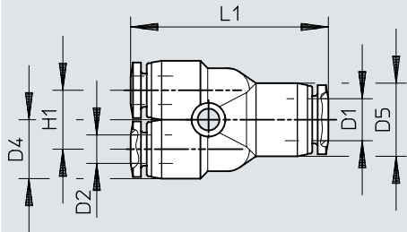
Dimensions – Union en Y QBM...T, réductrice
