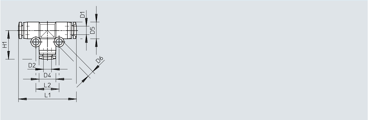
Dimensions – Union en T QBMT-...T, réductrice
