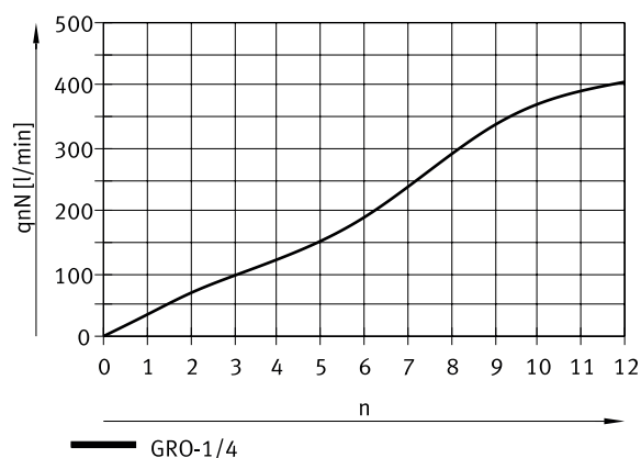
Portata nominale normale qnN a 6 → 5 bar in funzione delle rotazioni n della vite (GRO-1/4)
