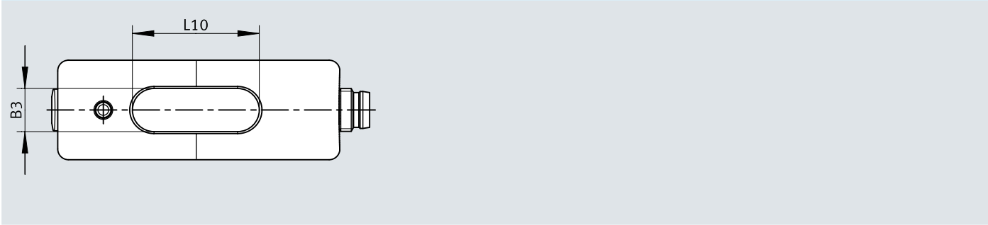
尺寸 - SPAF-...-L-...
