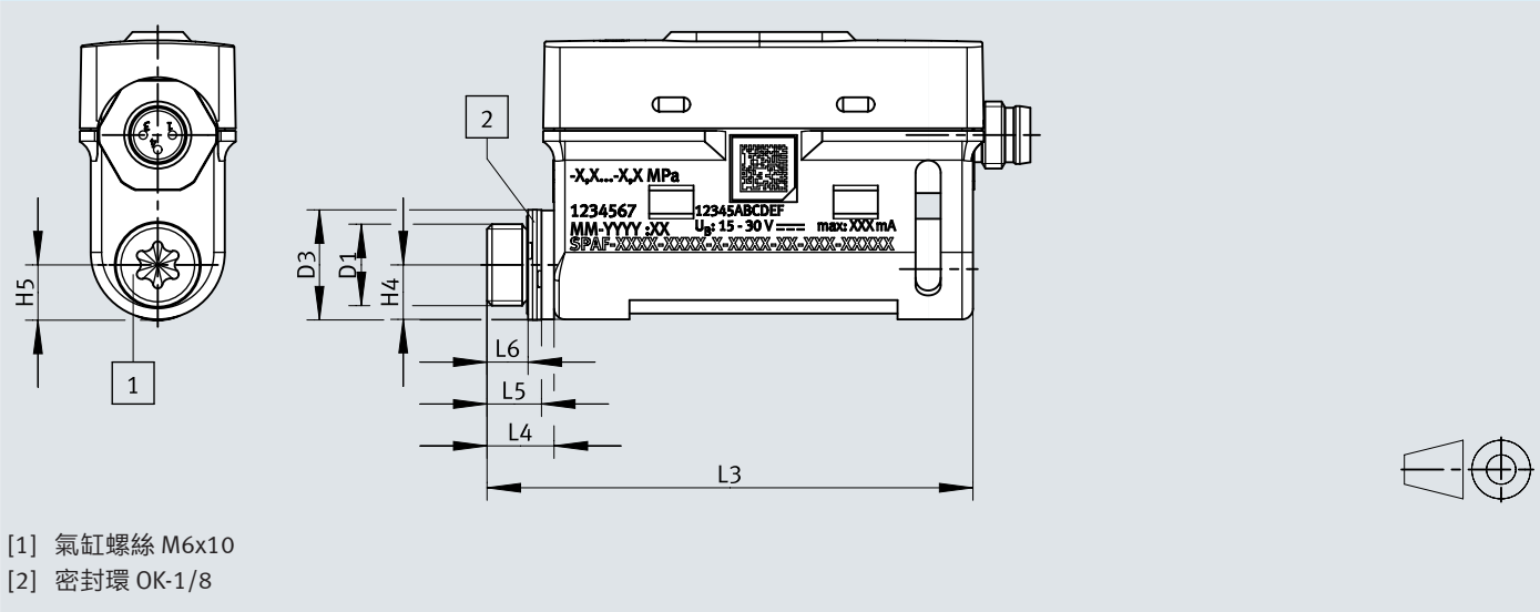
尺寸 – SPAF-...-G18M-...
