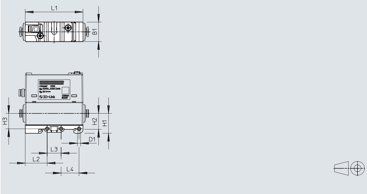
尺寸 – H 型導軌安裝件 SAMH-FH-H
