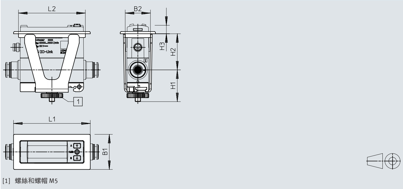
尺寸 – 前面板安裝套件 SAMH-FH-F
