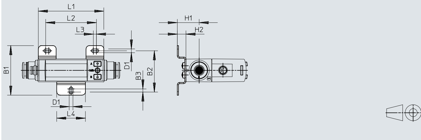
尺寸 – 牆面安裝元件 SAMH-FH-W
