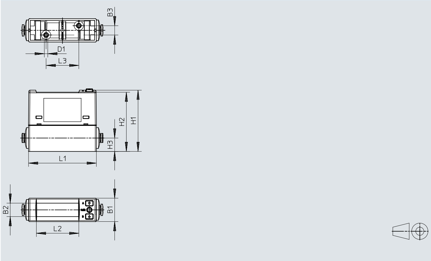
尺寸 - SFAH-...
