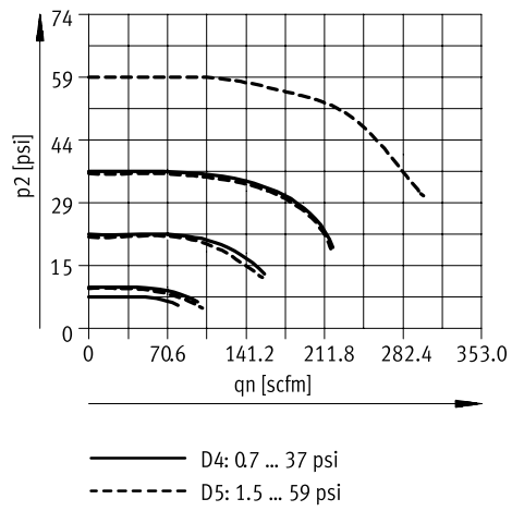
Caudal normal q_n en función de la presión de salida p_2 ( p_1 = 147 \text{ psi} ) – MS6N-LRPB-1/2
