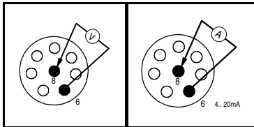
Fig. 21: Medidor de tensión Fig. 22: Medidor de corriente
