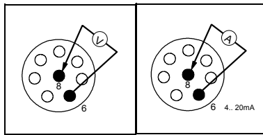
Bild 21: Spannungsmessgerät Fig. 21: Voltage measuring instrument Bild 22: Strommessgerät Fig. 22: Current measuring instrument
