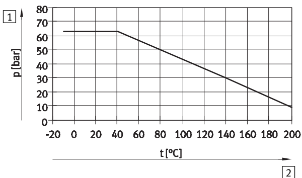
Fig. 5 Druck – Temperatur-Diagramm
