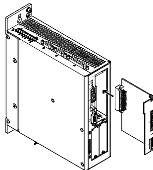
Fig. 3.1 Montage / Demontage
