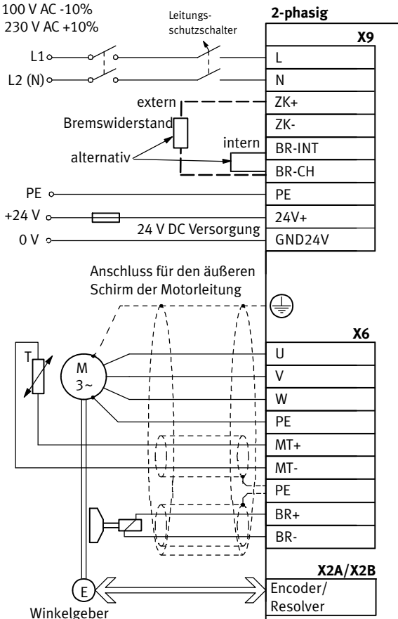
Fig. 4.2 CMMP-AS-...-3A-M3: Anschluss 2-phasig L1/L2 an die Versorgungsspannung und den Motor
