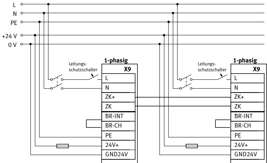
Fig. 4.6 Beispiel Zwischenkreiskopplung mit gemeinsamer Versorgung 1-phasig
